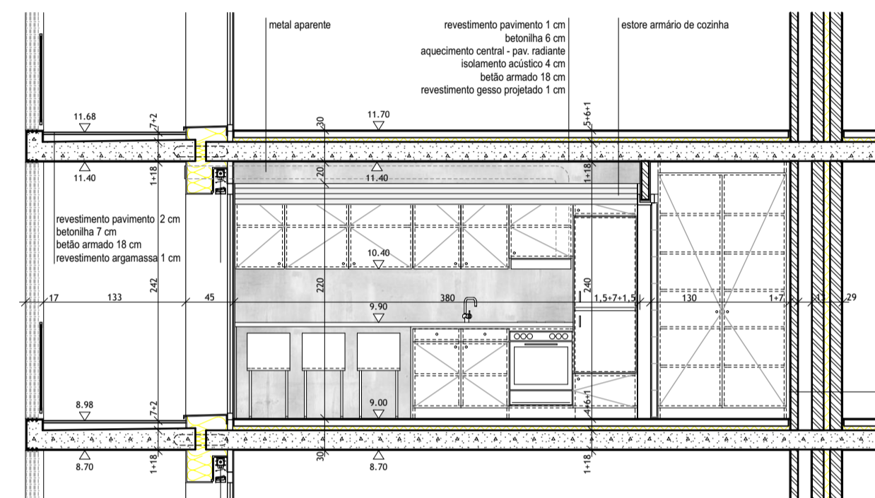
Corte F-F' 1/50
