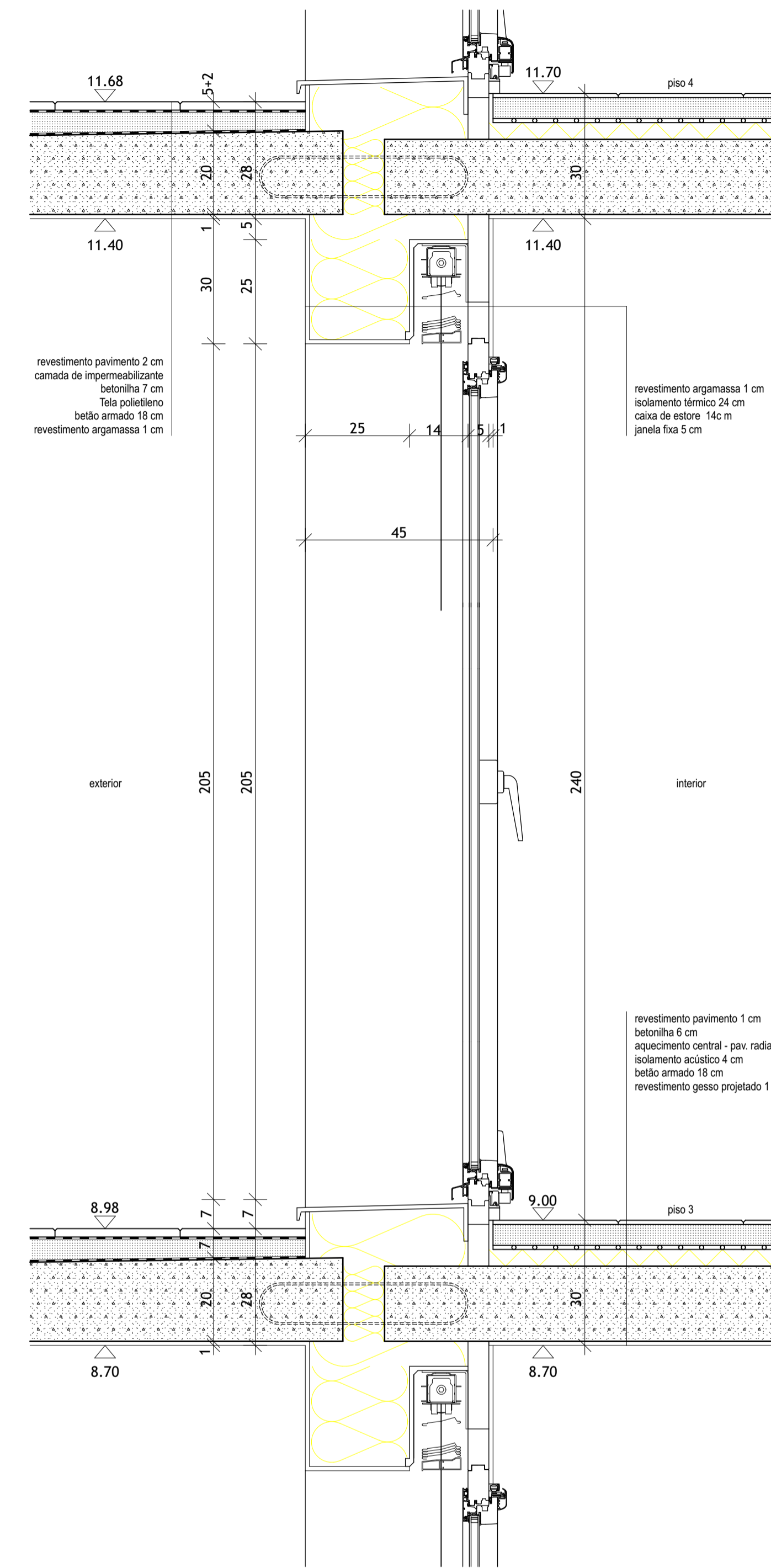
Corte detalhado do vão exterior 1/10
