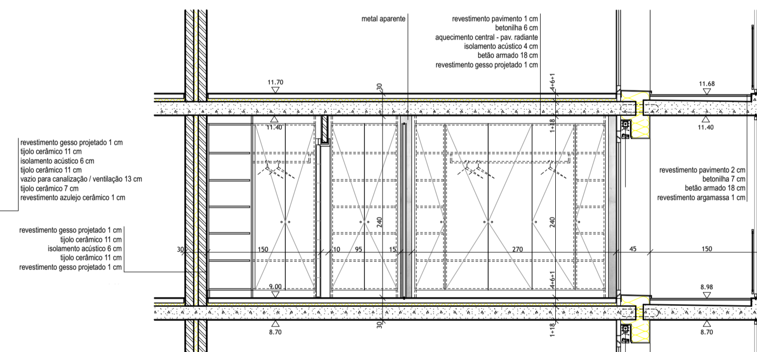
Corte I-I' 1/50
