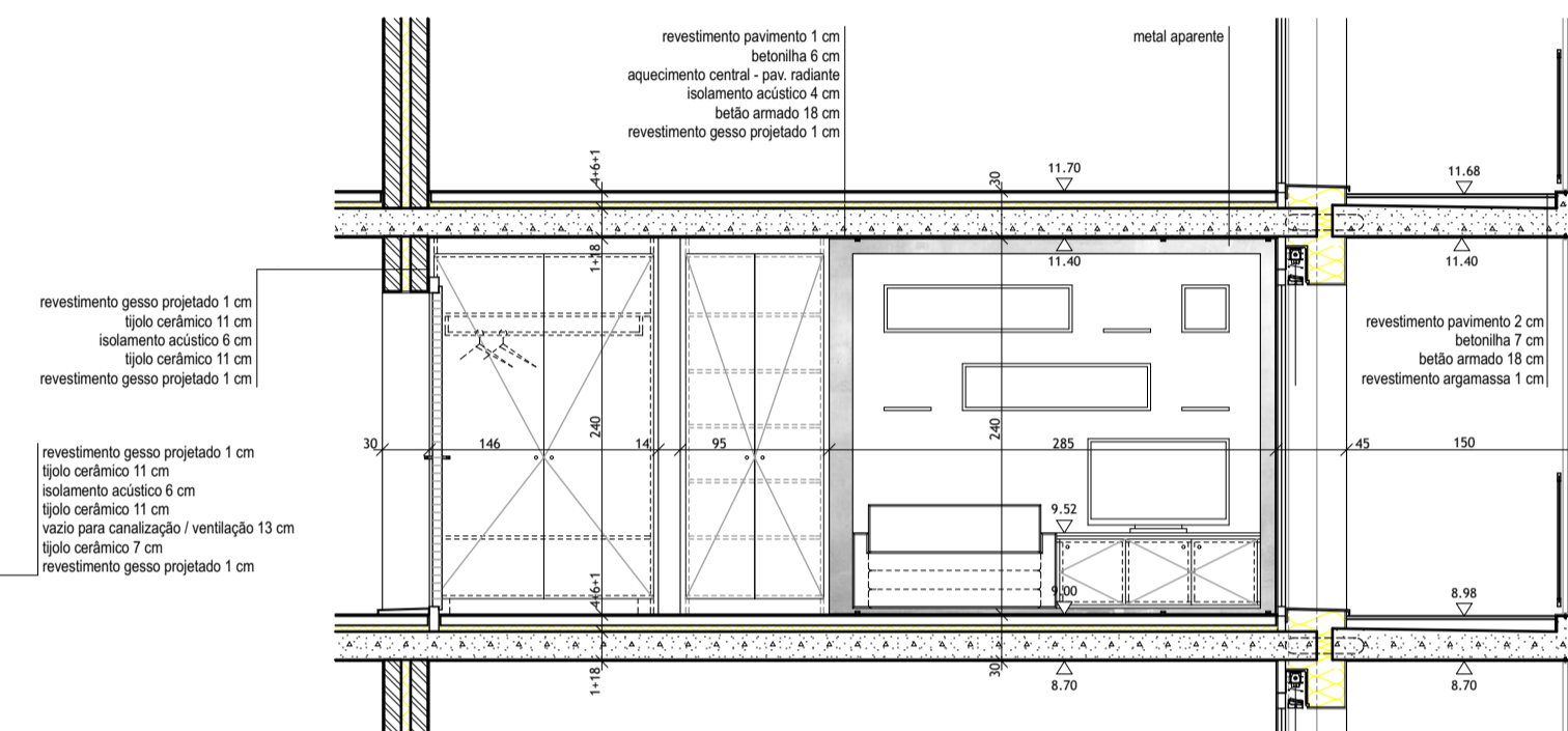
Corte G-G' 1/50
