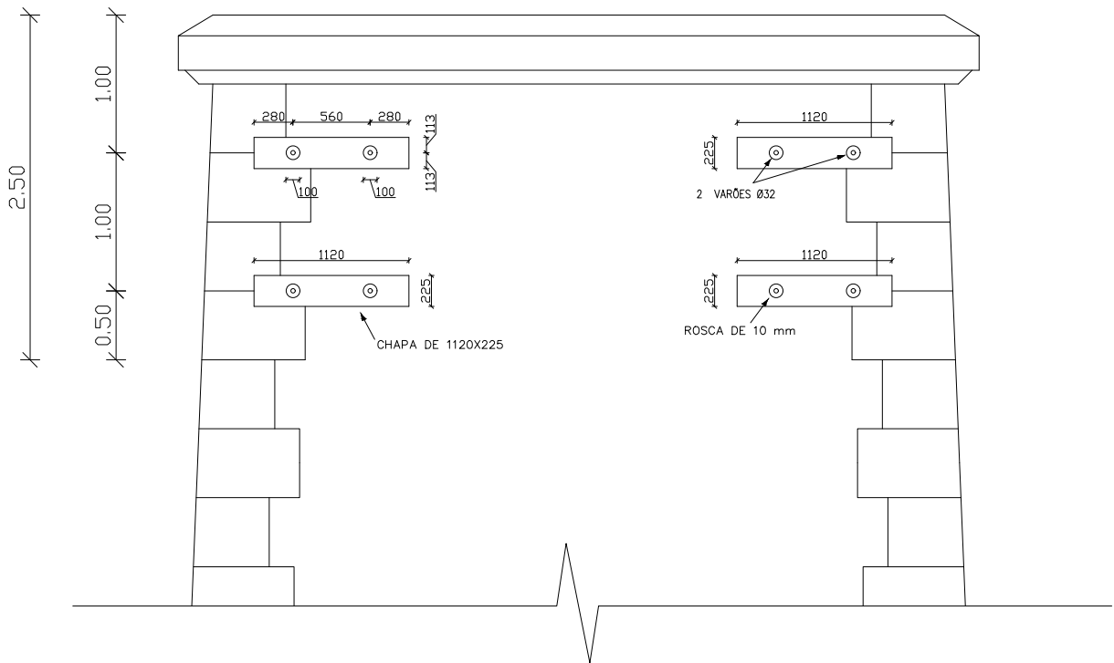
ALÇADO FRONTAL DO PILAR PRINCIPAL
