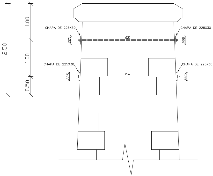
ALÇADO LATERAL DO PILAR PRINCIPAL
