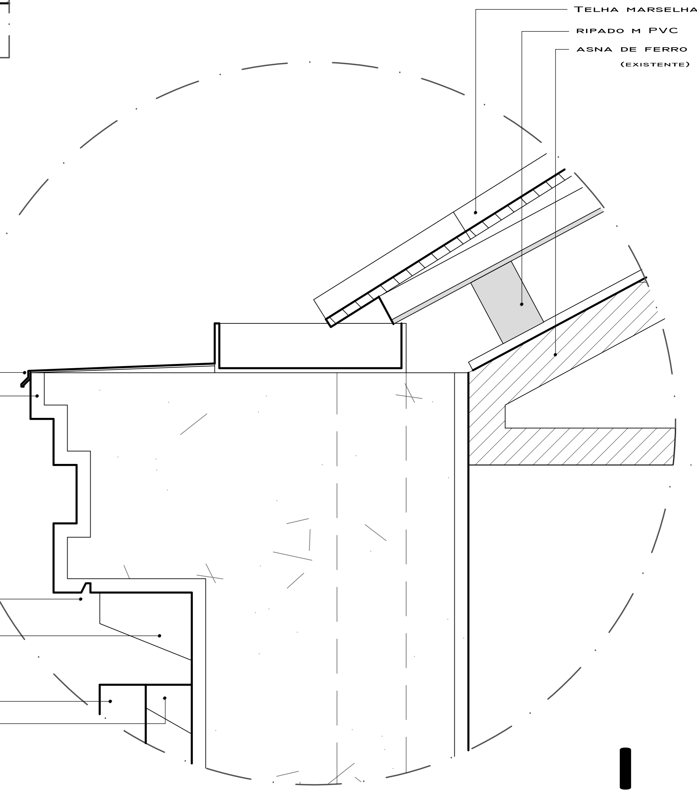
SECÇÃO TRANSVERSAL
