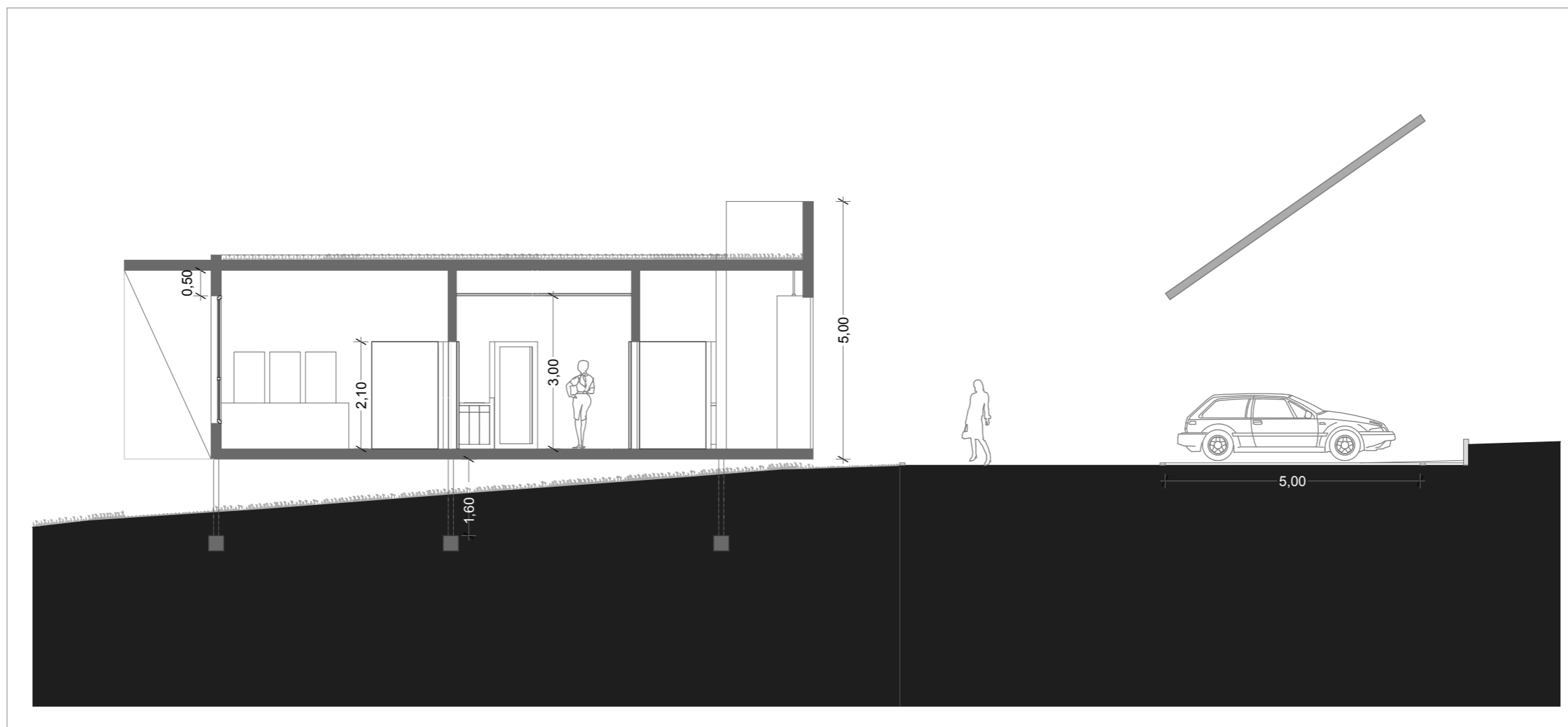
Corte B
