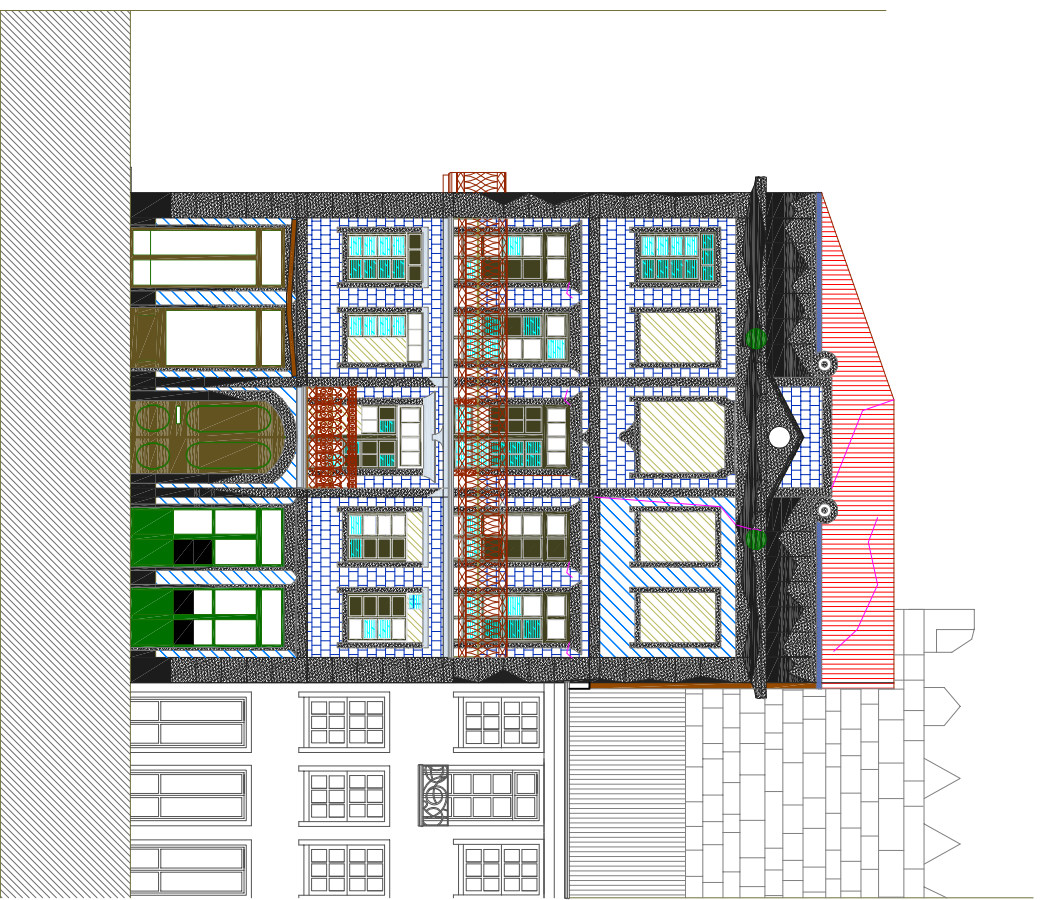
ALÇADO PRINCIPAL
