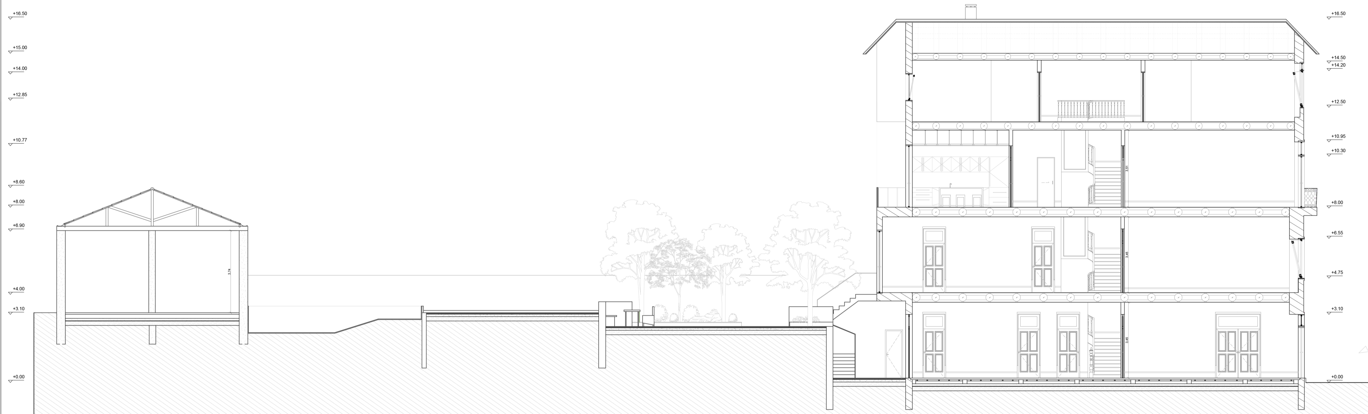
Corte longitudinal: A 01
