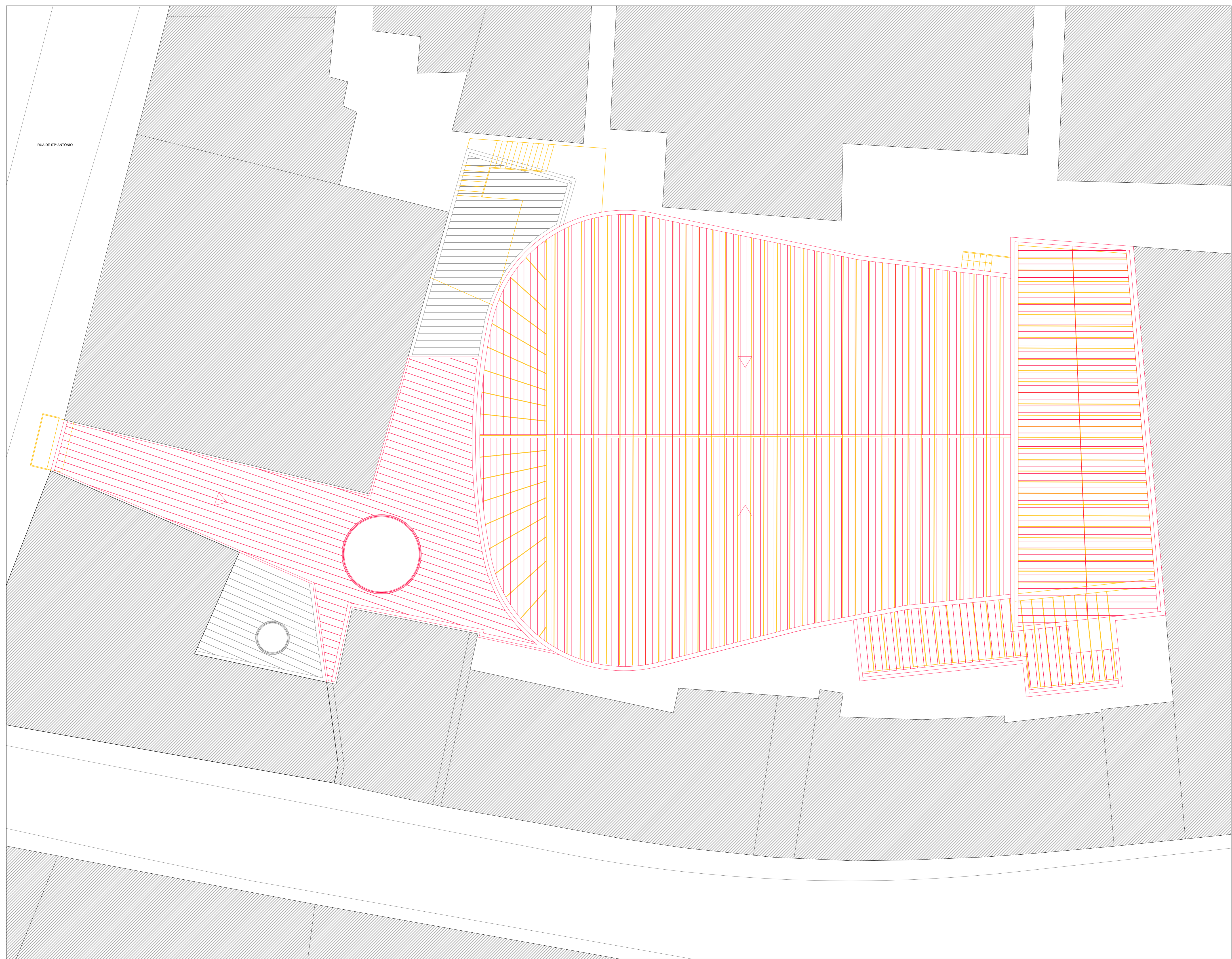
PLANTA DA COBERTURA (NÍVEL DA COTA 20,00)
