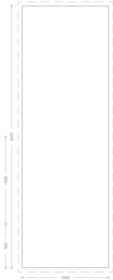
Imagem 299 - Levantamento gráfico da Janela V10 - Frente - Escala 1:25
