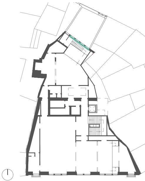
Imagem 297 - Localização da Janela V10 na planta de projeto - Escala 1:500
