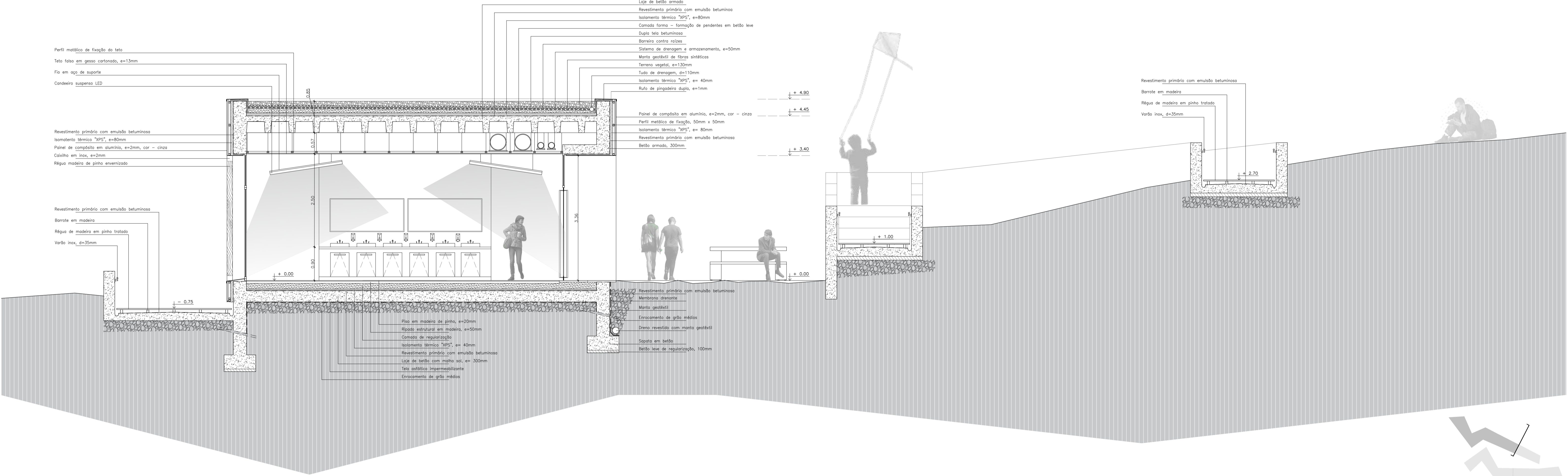
Corte I - Transversal A Caminho de Fátima. Conjunto multifuncional de apoio ao peregrino Dissertação de Mestrado - Universidade da Beira Interior Fábio Pereira Frazão - Nº 31222
