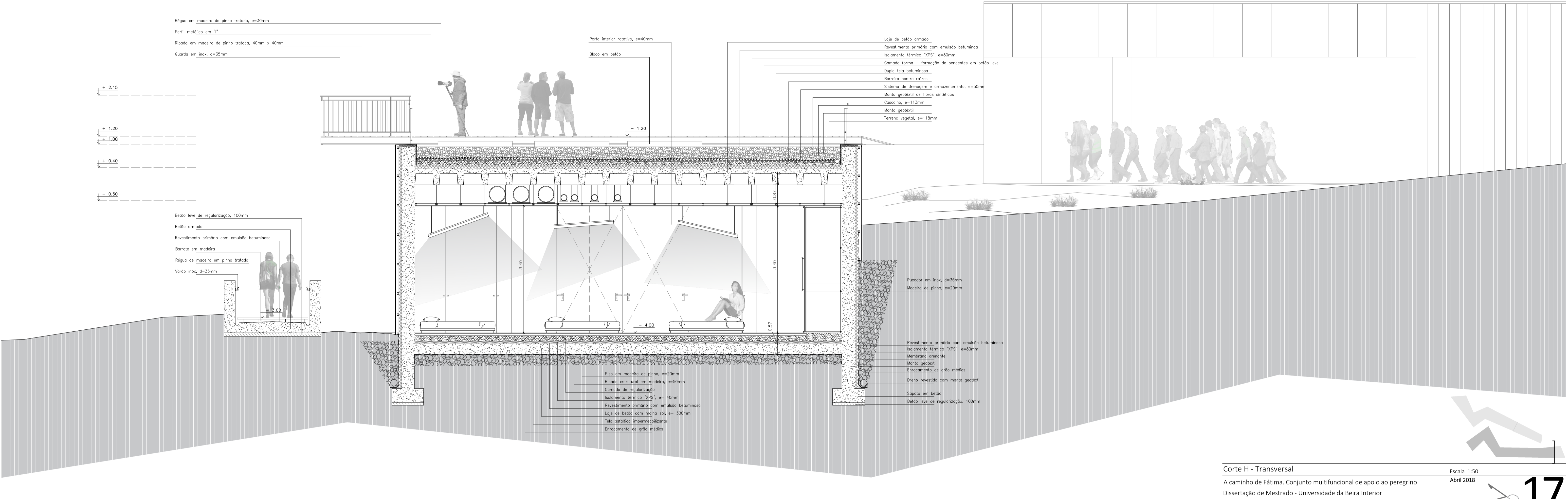
Corte G - Transversal A Caminho de Fátima. Conjunto multifuncional de apoio ao peregrino Dissertação de Mestrado - Universidade da Beira Interior Fábio Pereira Frazão - Nº 31222
