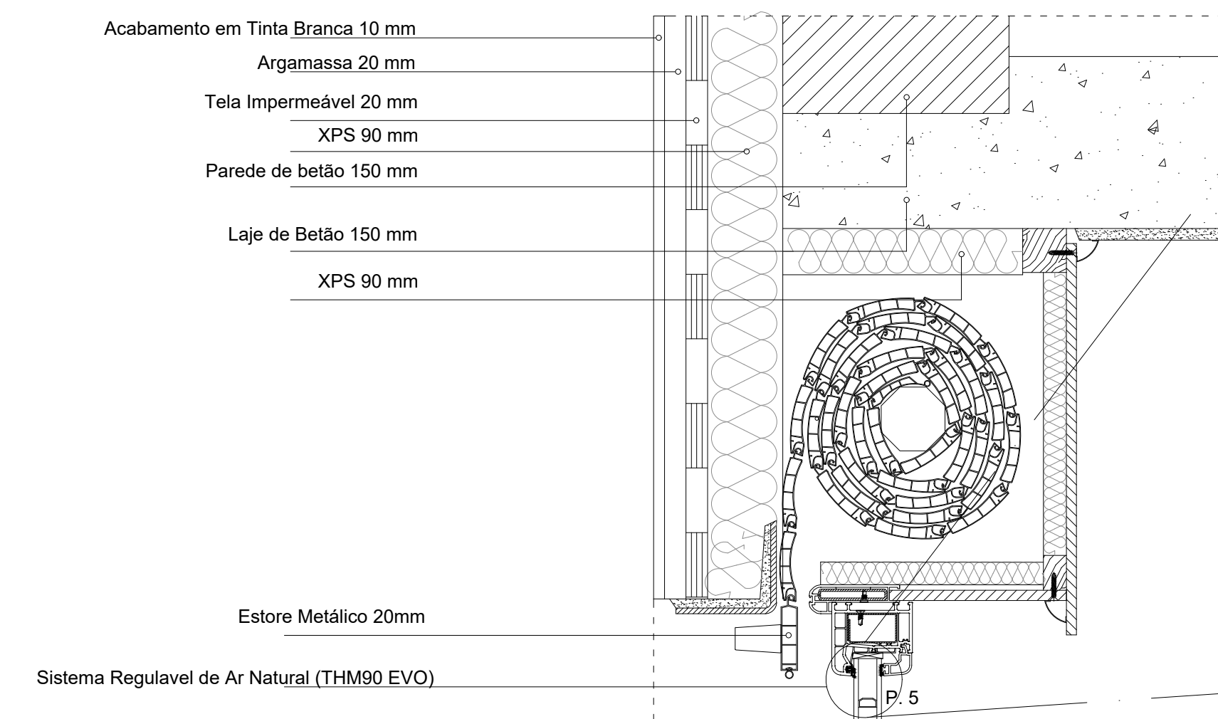
Pormenor 4 - opção 2
