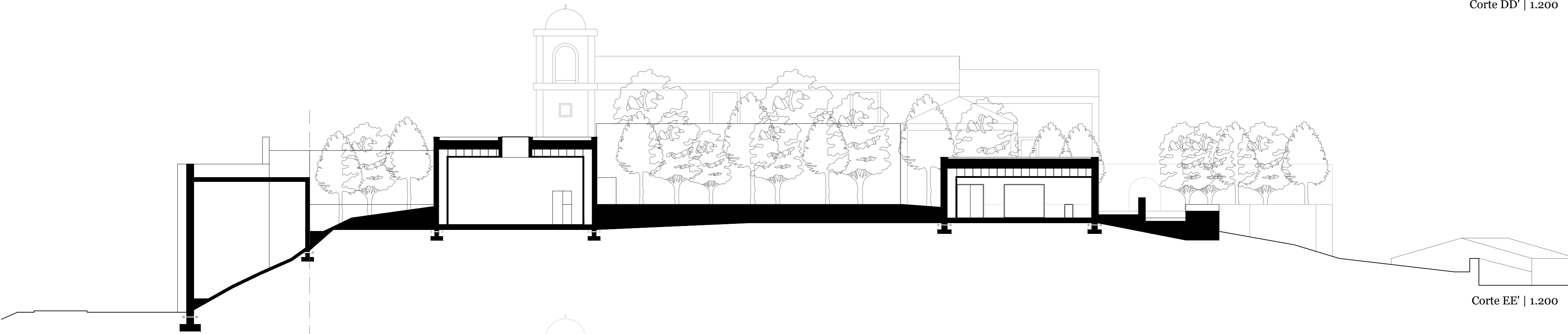
Corte DD' | 1.200
