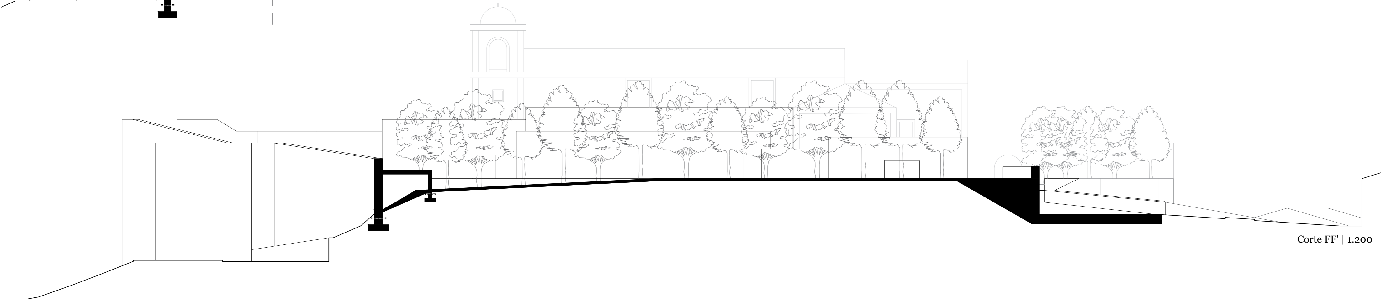
Corte EE' | 1.200
