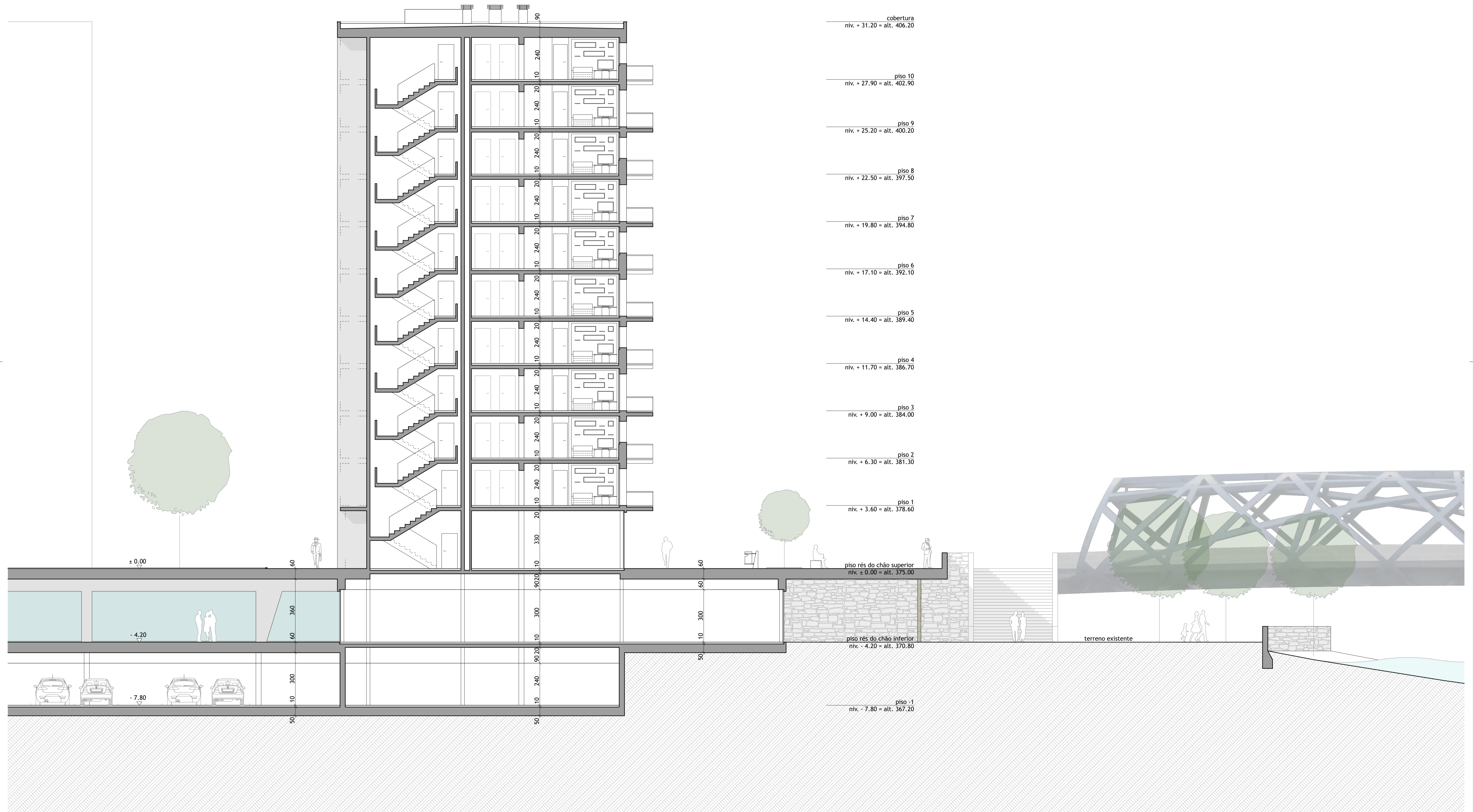
Corte B-B' 1/100
