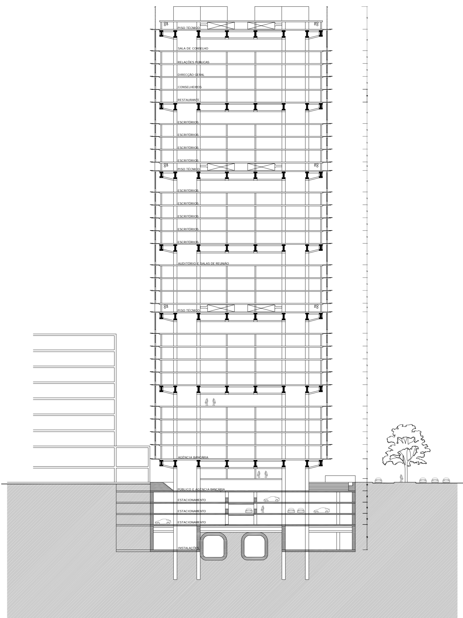
Corte transversal
