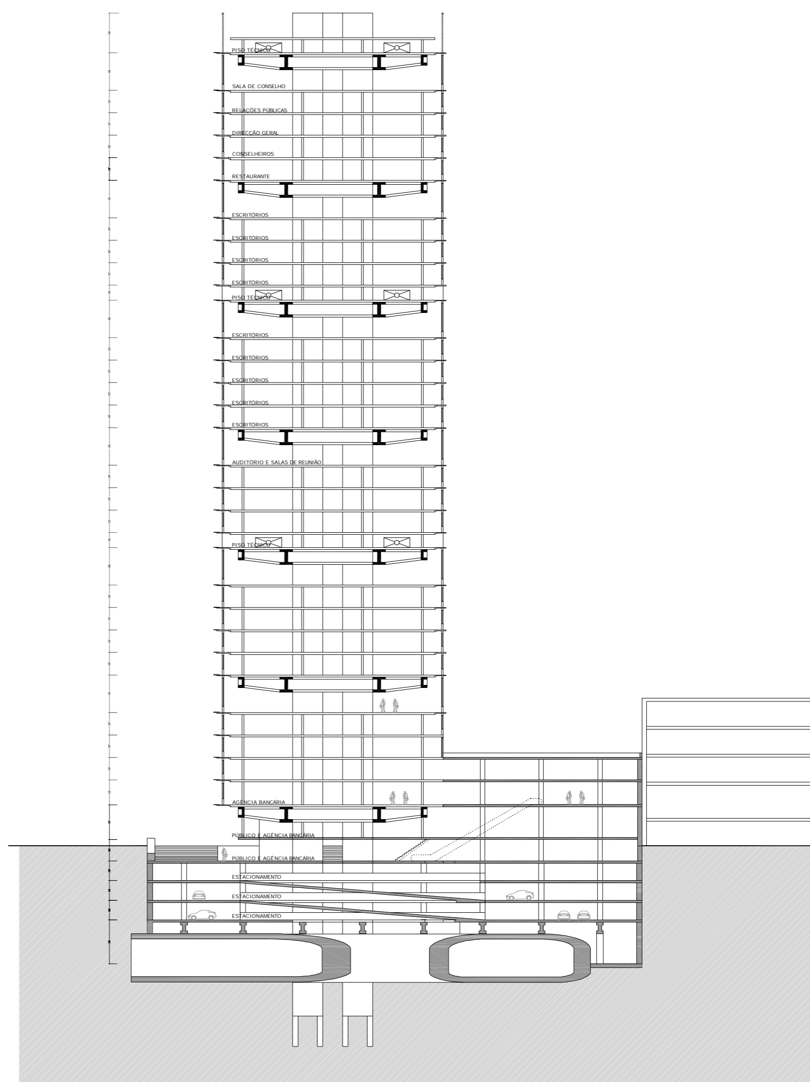
Corte longitudinal
