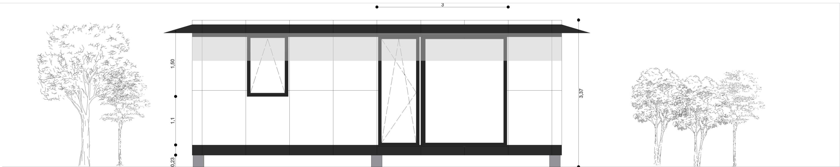
ALÇADO POENTE
