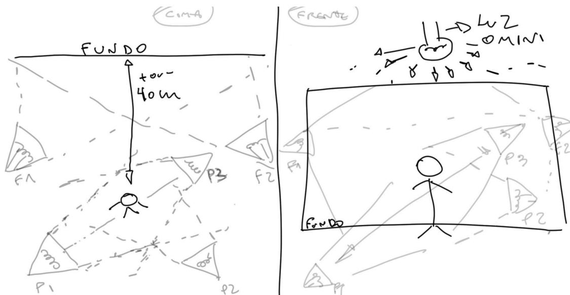
Figura 63: Esboço de set up de iluminação.
