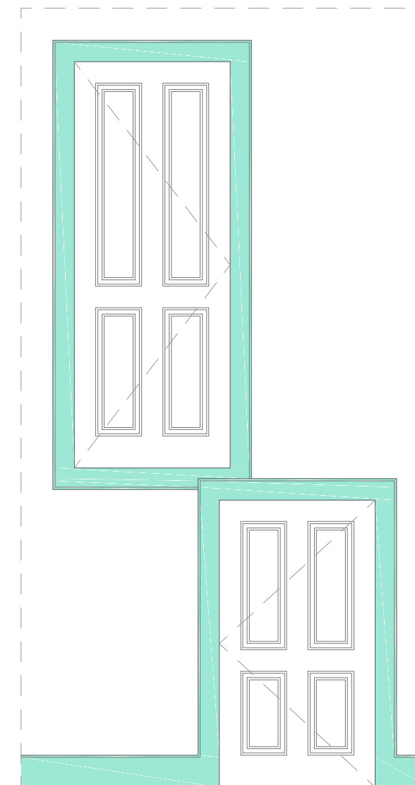
Imagem 244 - Levantamento gráfico a cores da Porta P7 e Porta P8 - Frente - Escala 1:25
