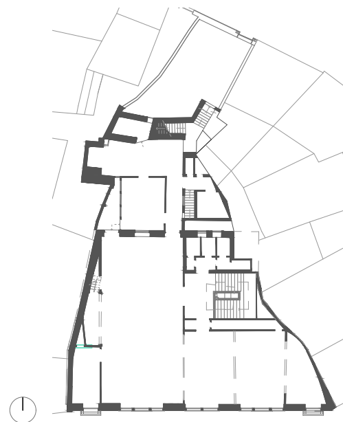
Imagem 242 - Localização da Porta P7 e Porta P8 na planta original - Escala 1:500
