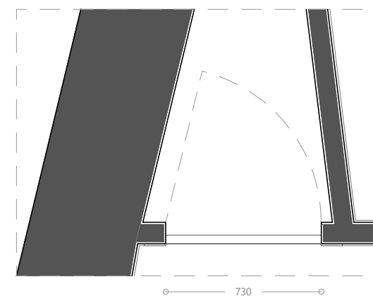
Imagem 245 - Levantamento gráfico da Porta P7 e Porta P8 - Planta - Escala 1:25
