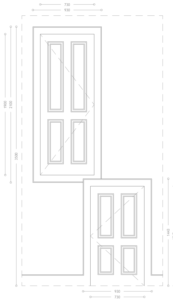
Imagem 243- Levantamento gráfico da Porta P7 e Porta P8 - Frente - Escala 1:25
