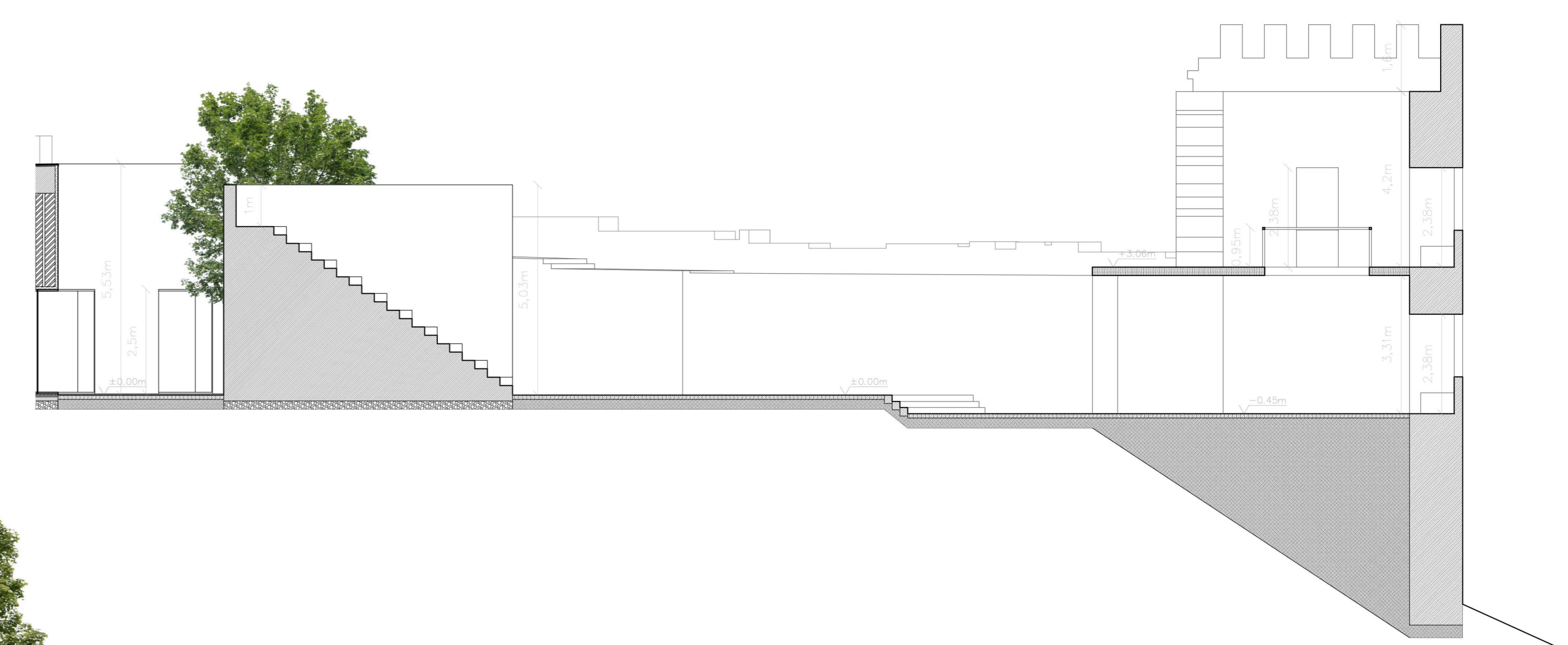
Corte JJ' | 1.100
