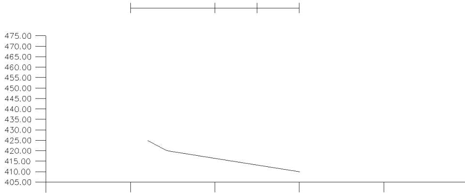
fig. 101 - Perfil CB_g1.11. Escala 1/3000.
