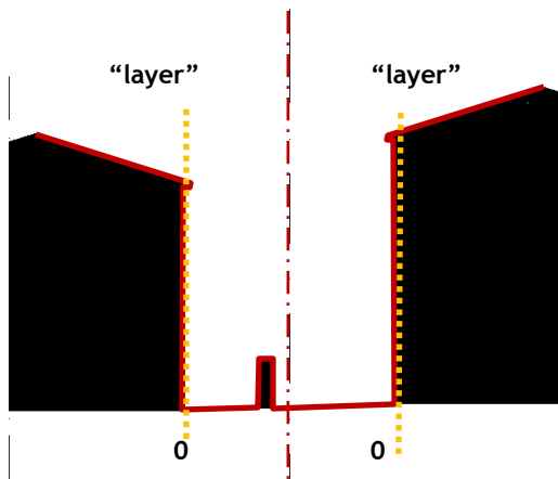
fig. 441 - G.pt16 - perfil transversal 16 - escala 1/500 (Rua do Amparo na Guarda - antiga Judiaria);
