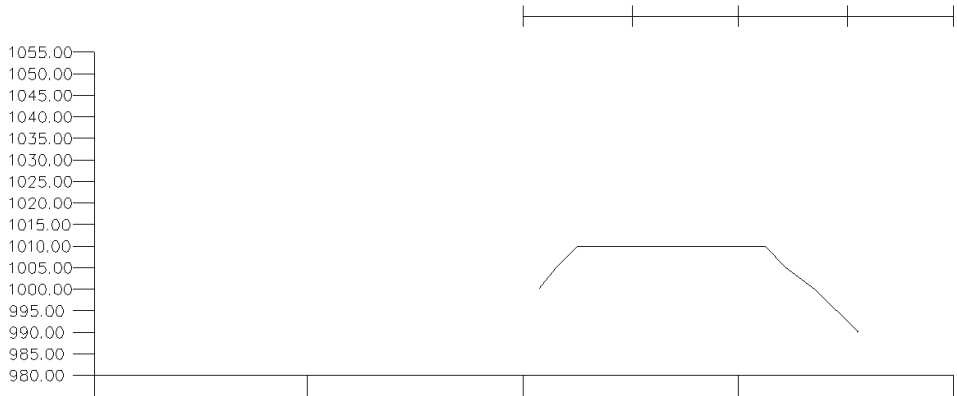
fig. 216 - Perfil G_g1.9. Escala 1/3000.
