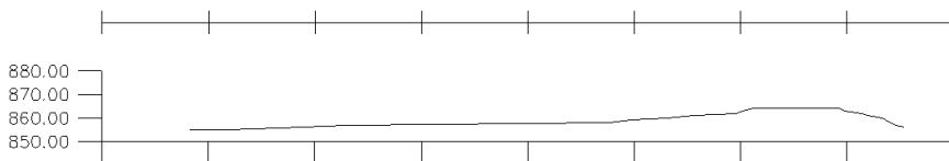
fig. 345 - Perfil T_g2.26. Escala 1/3000.
