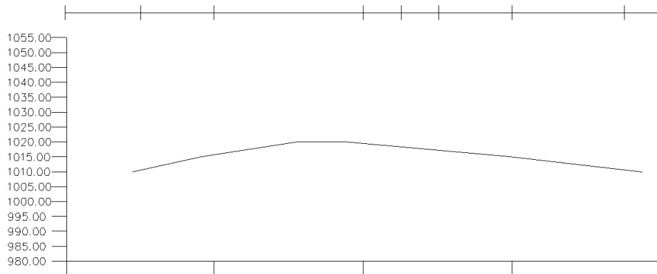
fig. 211 - Perfil G_g1.4. Escala 1/3000.
