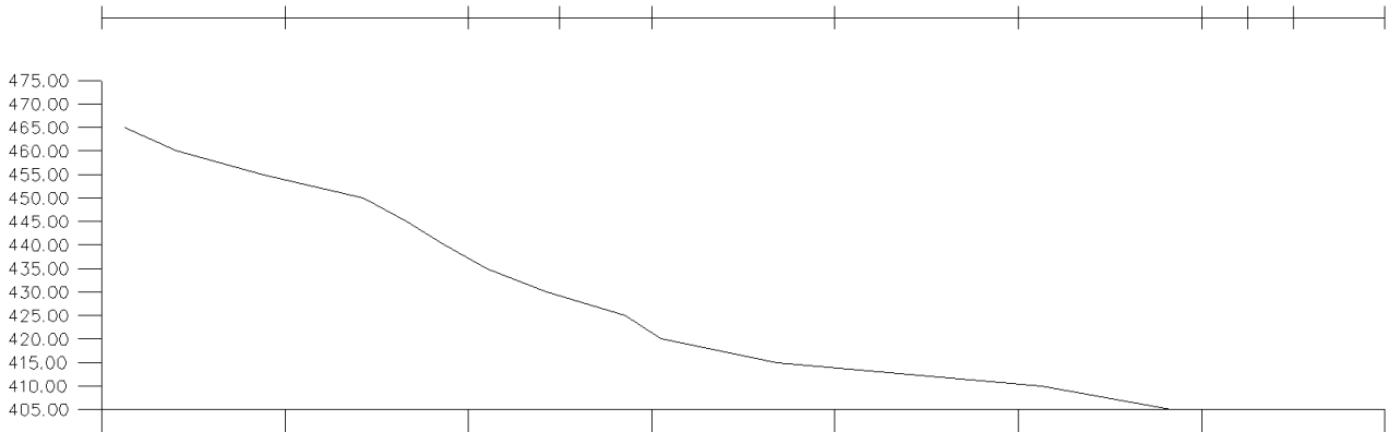
fig. 151 - Perfil CB_g3.15. Escala 1/3000.
