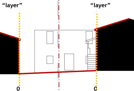
fig. 437 - G.pt12 - perfil transversal 12 - escala 1/500 (Rua do Amparo na Guarda - antiga Judiaria);
