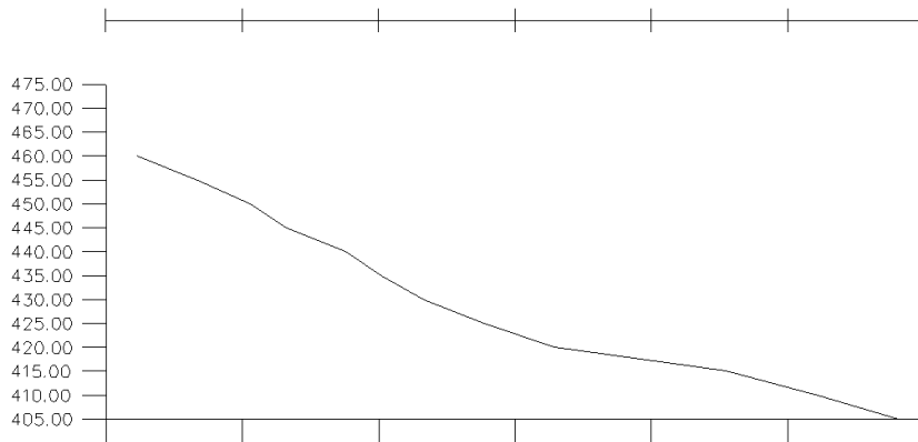
fig. 122 - Perfil CB_g2.12. Escala 1/3000.
