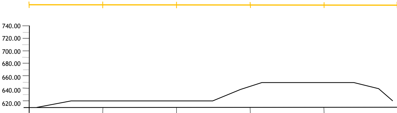
fig. 07 - Perfil C_g1.1 orientado a sul/norte. Escala 1/3000.
