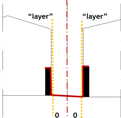
fig. 411 - CB.pt2 - perfil transversal 2 - escala 1/500 (Rua do Muro em Castelo Branco - antiga Judiaria);
