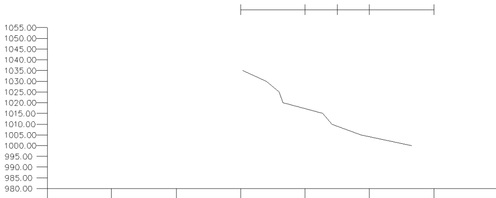
fig. 238 - Perfil G_g2.8. Escala 1/3000.
