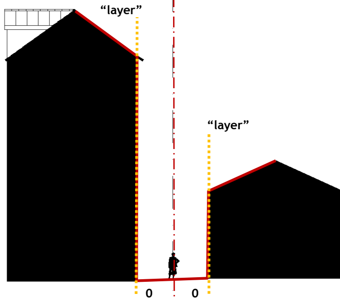
fig. 405 - C.pt23 - perfil transversal 23 - escala 1/500 (Rua da Alegria na Covilhã - antiga Judiaria);
