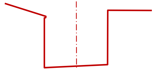
fig. 433 - G.pt8 - perfil transversal 8 - escala 1/500 (Rua do Amparo na Guarda - antiga Judiaria);
