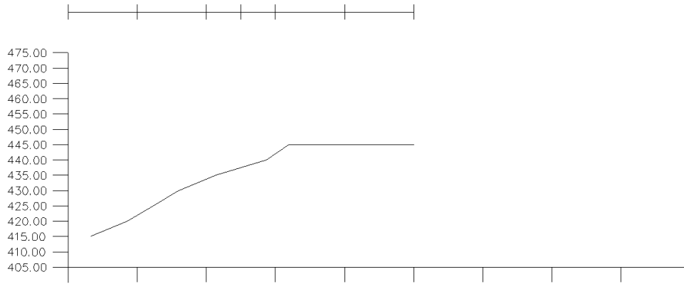
fig. 148 - Perfil CB_g3.13. Escala 1/3000.
