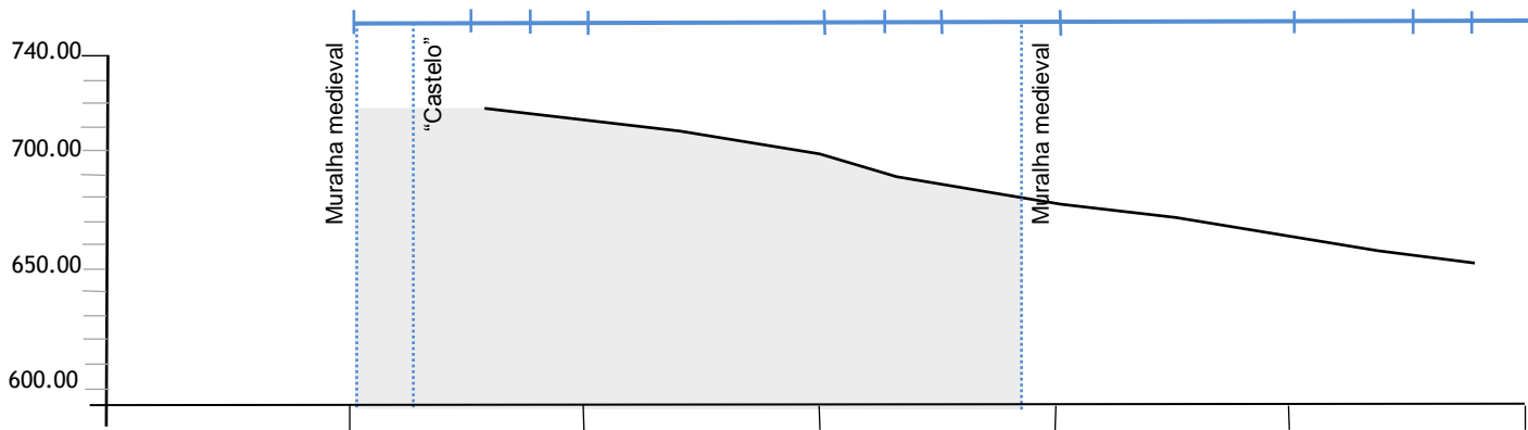
fig. 48 - Perfil C_g2.9 orientado a sul/norte. Escala 1/3000.
