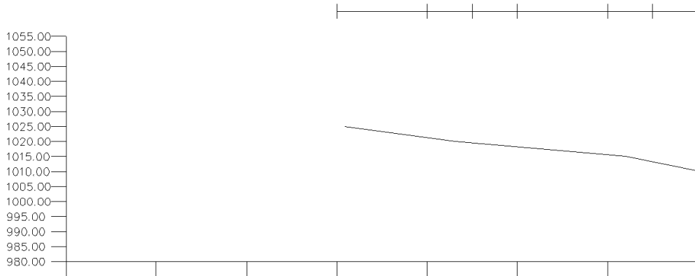
fig. 232 - Perfil G_g2.2. Escala 1/3000.
