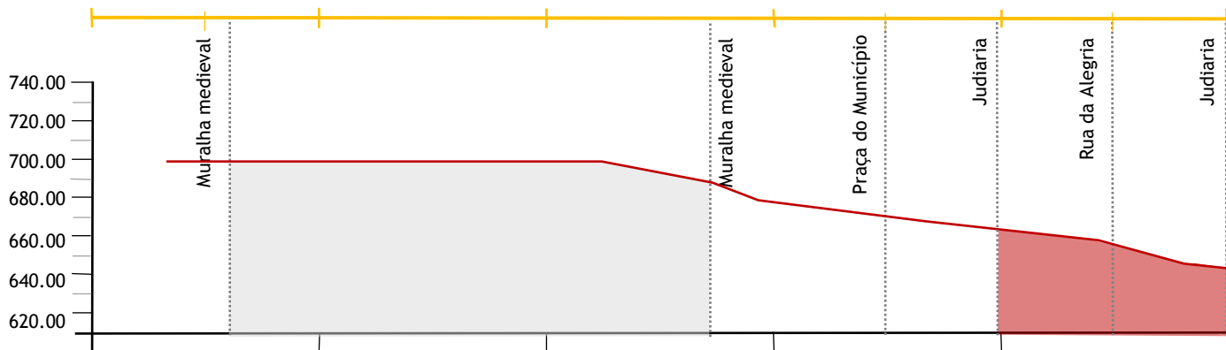
fig. 18 - Perfil C_g1.12 orientado a sul/norte. Escala 1/3000.
