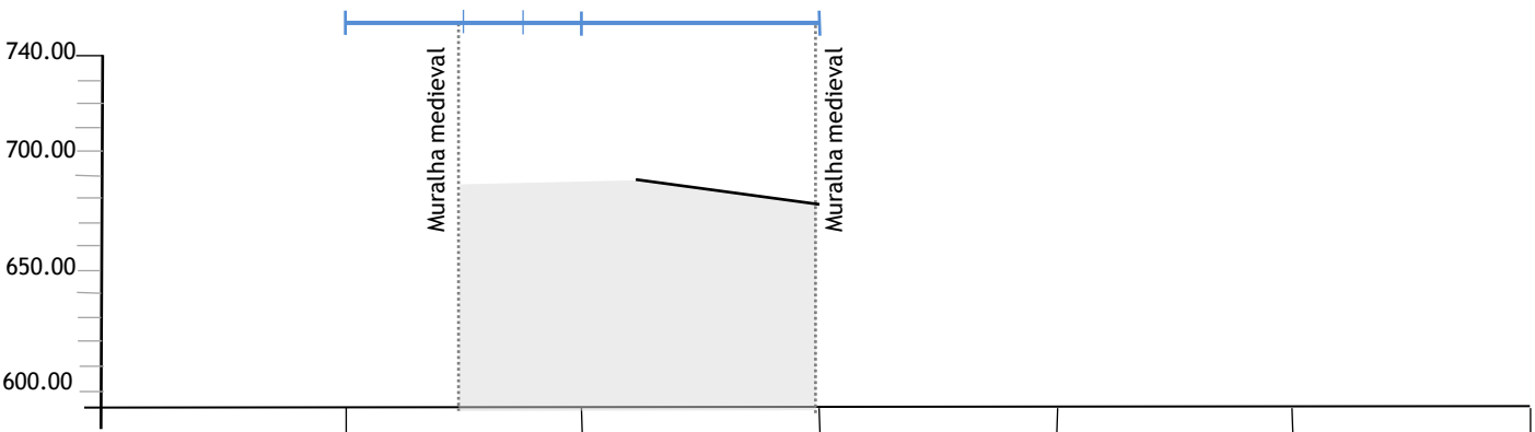
fig. 43 - Perfil C_g2.4 orientado a sul/norte. Escala 1/3000.
