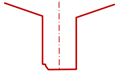
fig. 417 - CB.pt8 - perfil transversal 8 - escala 1/500 (Rua do Muro em Castelo Branco - antiga Judiaria);
