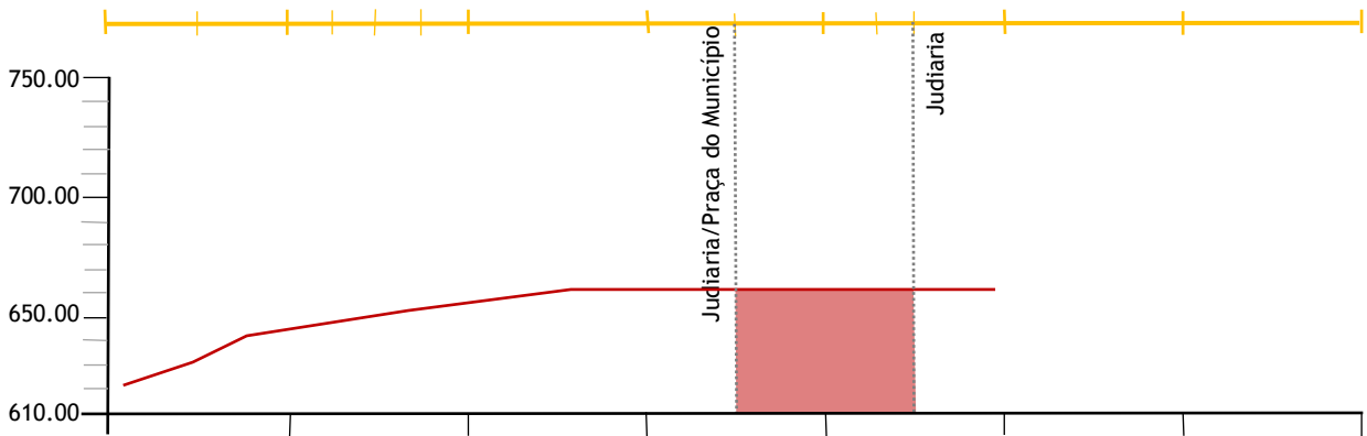
fig. 34 - Perfil C_g1.27 orientado a nasceste/poente. Escala 1/3000.
