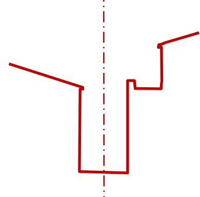
fig. 461 - T.pt5 - perfil transversal 5 - escala 1/500 (Rua da Alegria em Trancoso - antiga Judiaria);
