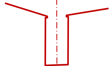
fig. 434 - G.pt9 - perfil transversal 9 - escala 1/500 (Rua do Amparo na Guarda - antiga Judiaria);
