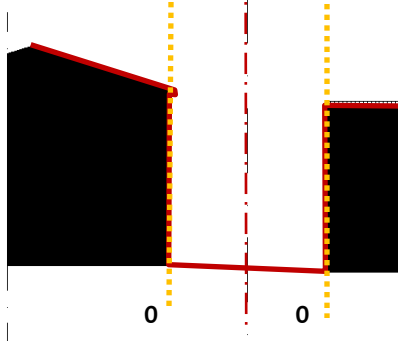
fig. 431 - G.pt6 - perfil transversal 6 - escala 1/500 (Rua do Amparo na Guarda - antiga Judiaria);
