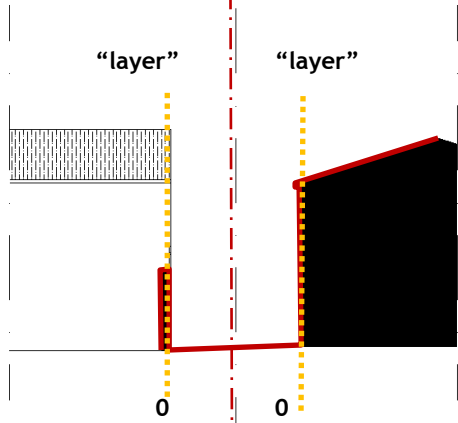
fig. 445 - G.pt20 - perfil transversal 20 - escala 1/500 (Rua do Amparo na Guarda - antiga Judiaria);
