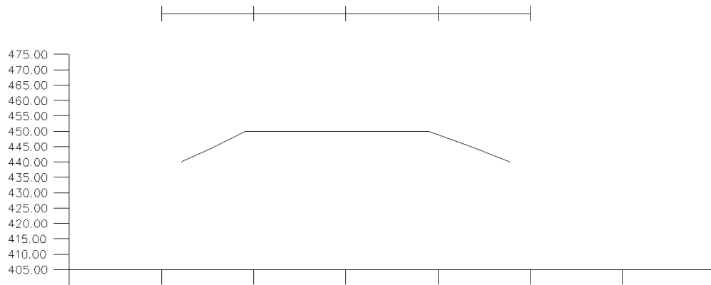
fig. 96 - Perfil CB_g1.7. Escala 1/3000.
