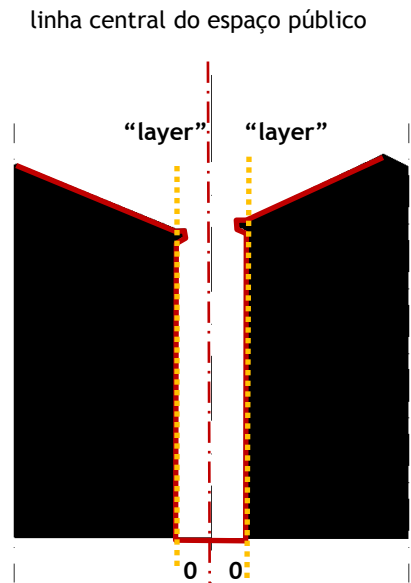
fig. 454 - T.pt1 - perfil transversal 1 escala 1/500 (Rua da Alegria em Trancoso - antiga Judiaria);
