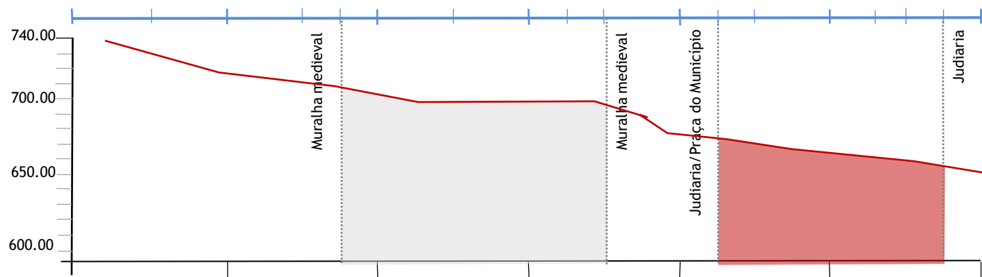
fig. 73 - Perfil C_g2.33 orientado a nascente/poente. Escala 1/3000.
