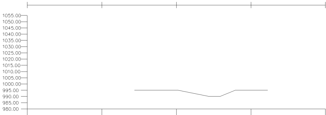
fig. 257 - Perfil G_g3.5. Escala 1/3000.
