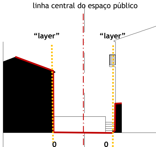
fig. 419 - CB.pt10 - perfil transversal 10 - escala 1/500 (Rua do Muro em Castelo Branco - antiga Judiaria);
