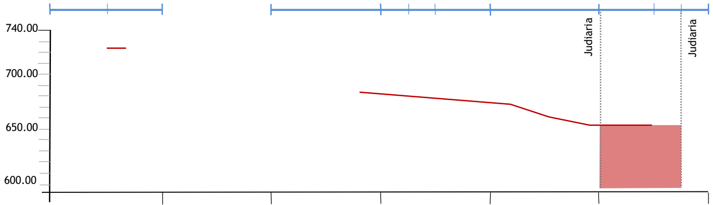
fig. 56 - Perfil C_g2.17 orientado a sul/norte. Escala 1/3000.
