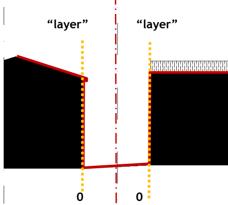
fig. 446 - G.pt21 - perfil transversal 21 - escala 1/500 (Rua do Amparo na Guarda - antiga Judiaria);
