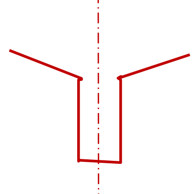
fig. 462 - T.pt6 - perfil transversal 6 - escala 1/500 (Rua da Alegria em Trancoso - antiga Judiaria);
