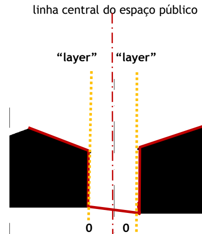
fig. 425 - CB.pt16 - perfil transversal 16 - escala 1/500 (Rua do Muro em Castelo Branco - antiga Judiaria);
