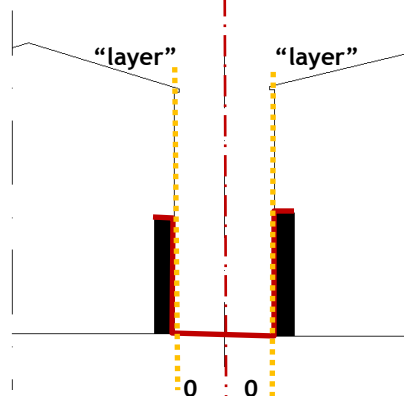
fig. 412 - CB.pt3 - perfil transversal 3 - escala 1/500 (Rua do Muro em Castelo Branco - antiga Judiaria).
