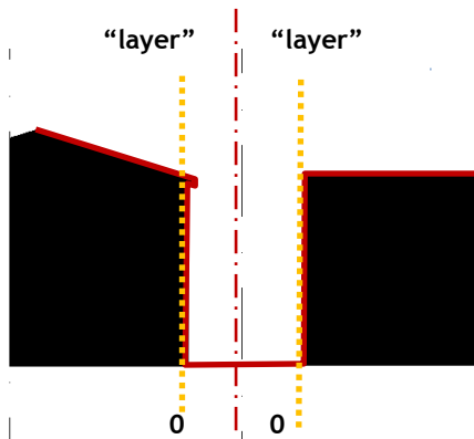
fig. 447 - G.pt22 - perfil transversal 22 - escala 1/500 (Rua do Amparo na Guarda - antiga Judiaria);
