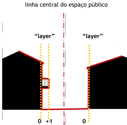
fig. 444 - G.pt19 - perfil transversal 19 - escala 1/500 (Rua do Amparo na Guarda - antiga Judiaria);
