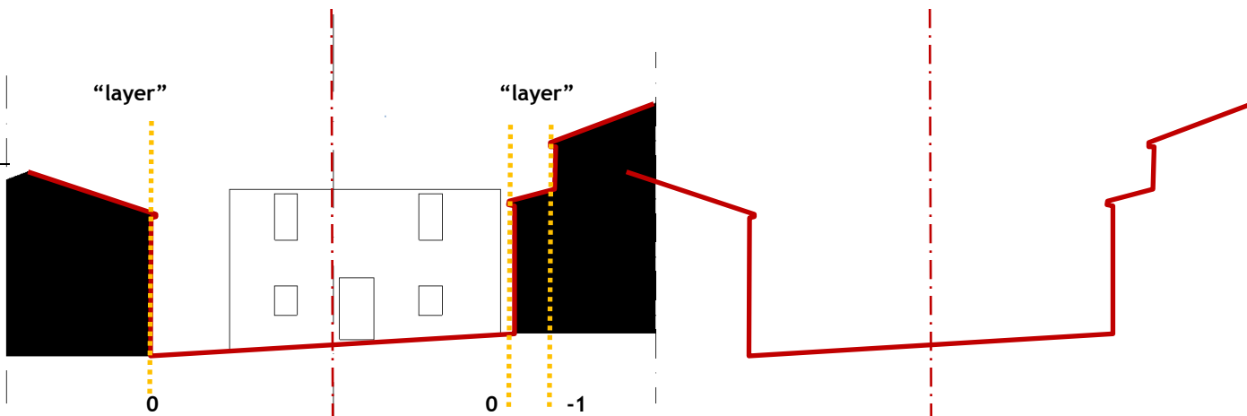
fig. 438 - G.pt13 - perfil transversal 13 - escala 1/500 (Rua do Amparo na Guarda - antiga Judiaria);
