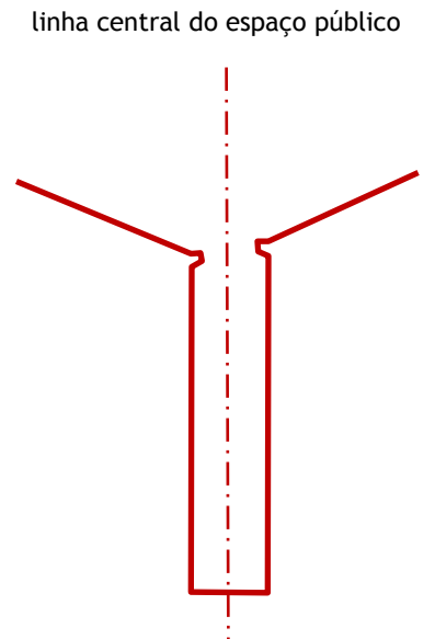
fig. 454 - T.pt1 - perfil transversal 1 escala 1/500 (Rua da Alegria em Trancoso - antiga Judiaria);
