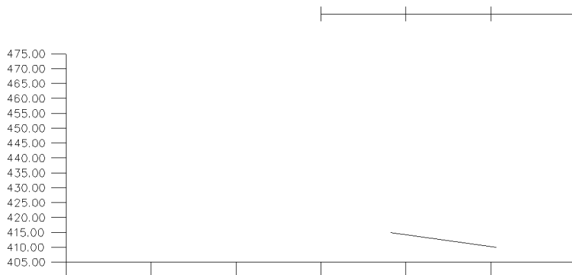
fig. 127 - Perfil CB_g2.17. Escala 1/3000.
