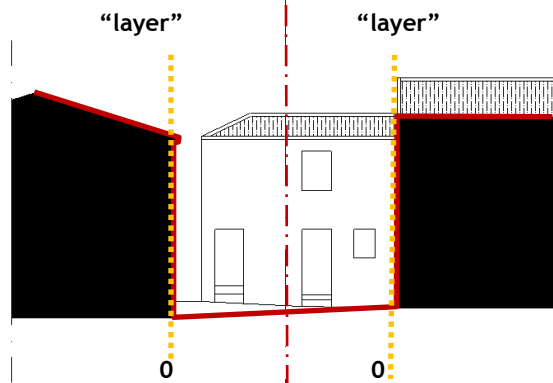
fig. 433 - G.pt8 - perfil transversal 8 - escala 1/500 (Rua do Amparo na Guarda - antiga Judiaria);
