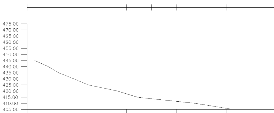
fig. 103 - Perfil CB_g1.13. Escala 1/3000.
