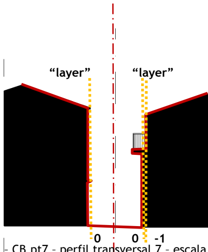
fig. 416 - CB.pt7 - perfil transversal 7 - escala 1/500 (Rua do Muro em Castelo Branco - antiga Judiaria);
