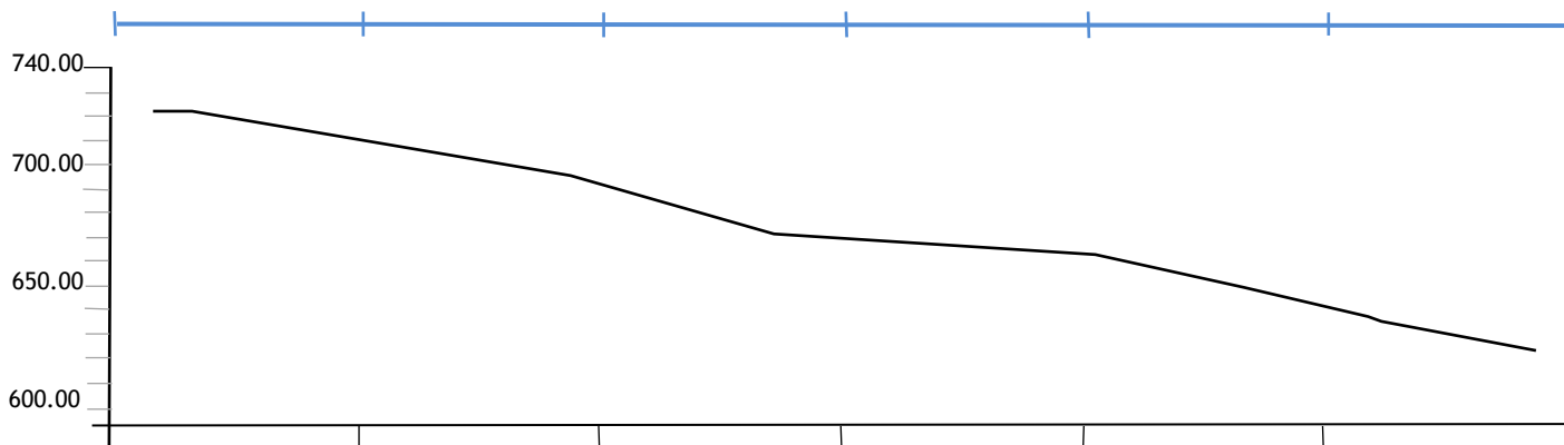
fig. 59 - Perfil C_g2.20 orientado a sul/norte. Escala 1/3000.
