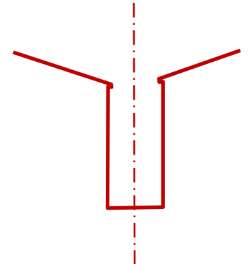
fig. 426 - G.pt1 - perfil transversal 1 - escala 1/500 (Rua do Amparo na Guarda - antiga Judiaria);
