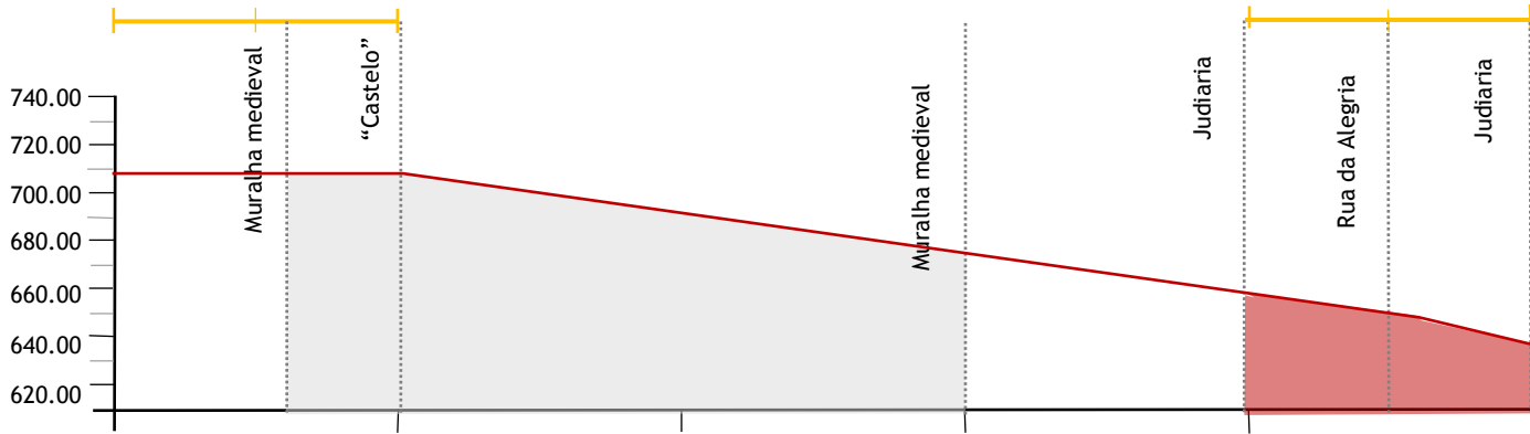
fig. 20 - Perfil C_g1.14 orientado a sul/norte. Escala 1/3000.
