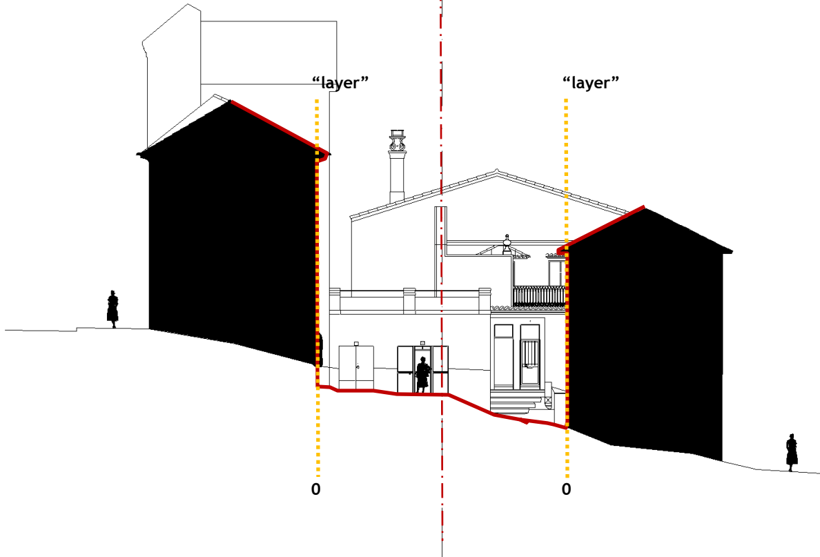
fig. 384 - C.pt2 - perfil transversal 2 - escala 1/500 (Rua da Alegria na Covilhã - antiga Judiaria).
