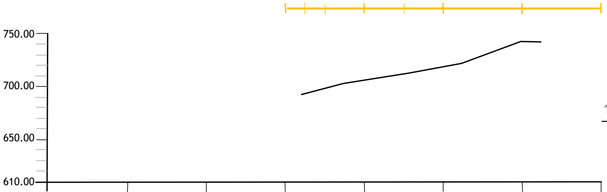
fig. 24 - Perfil C_g1.17 orientado a nasceste/ponte. Escala 1/3000.
