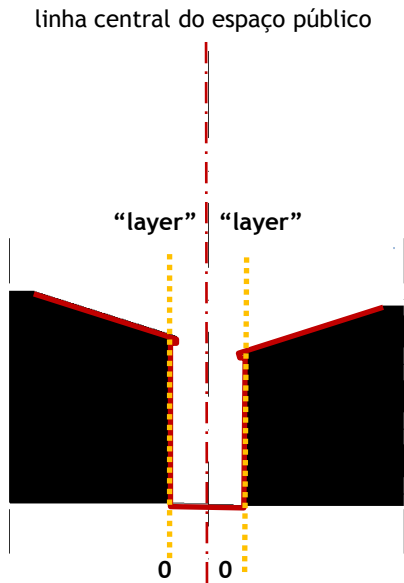
fig. 460 - T.pt4 - perfil transversal 4 - escala 1/500 (Rua da Alegria em Trancoso - antiga Judiaria);
