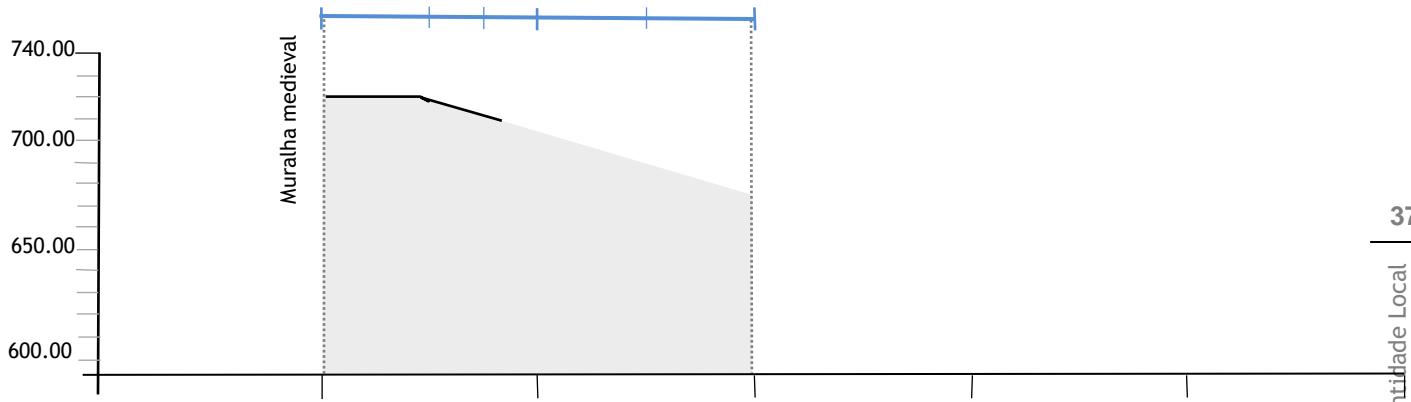
fig. 71 - Perfil C_g2.31 orientado a nascente/poente. Escala 1/3000.
