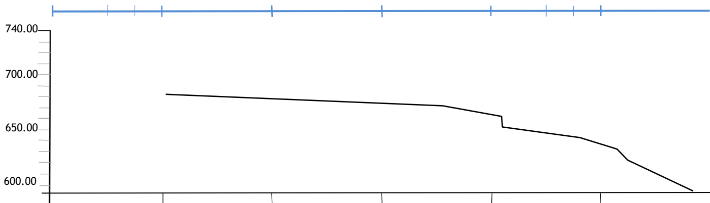
fig. 62 - Perfil C_g2.22 orientado a nascente/poente. Escala 1/3000.
