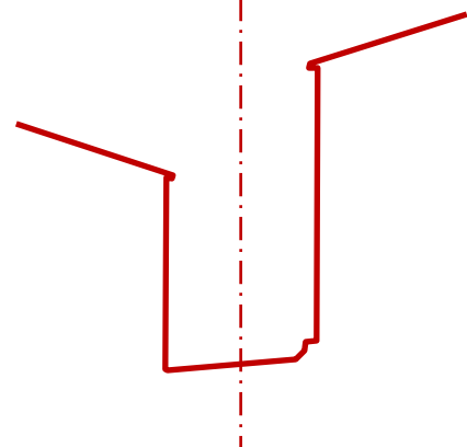
fig. 442 - G.pt17 - perfil transversal 17 - escala 1/500 (Rua do Amparo na Guarda - antiga Judiaria);
