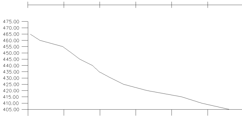
fig. 125 - Perfil CB_g2.15. Escala 1/3000.
