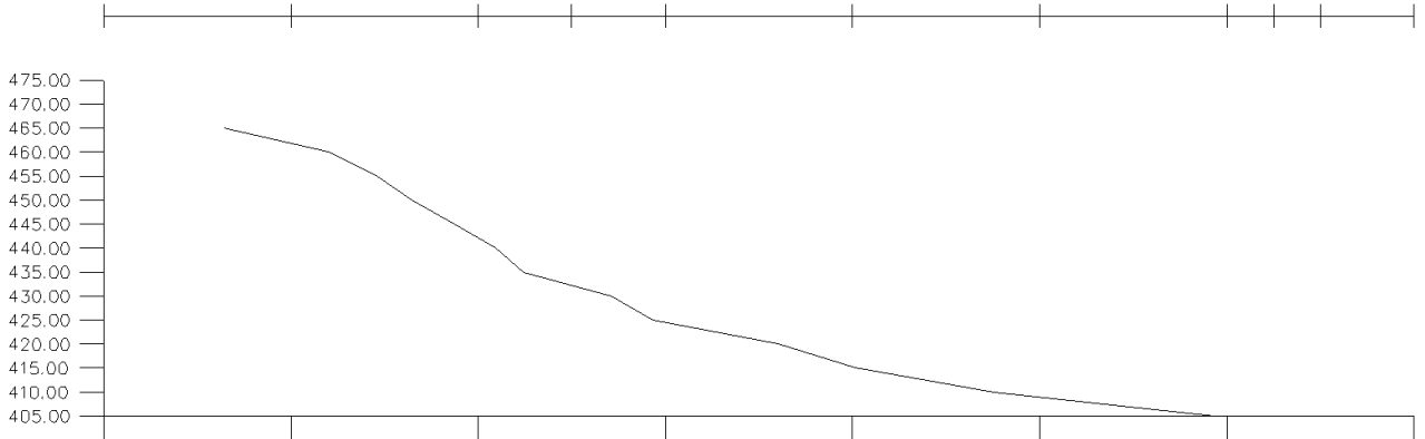
fig. 154 - Perfil CB_g3.18. Escala 1/3000.
