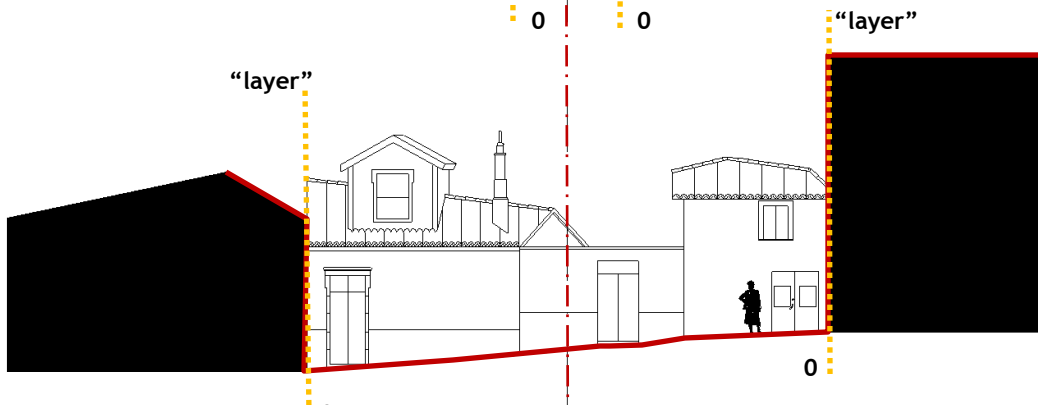
fig. 400 - C.pt18 - perfil transversal 18 - escala 1/500 (Rua da Alegria na Covilhã - antiga Judiaria);
