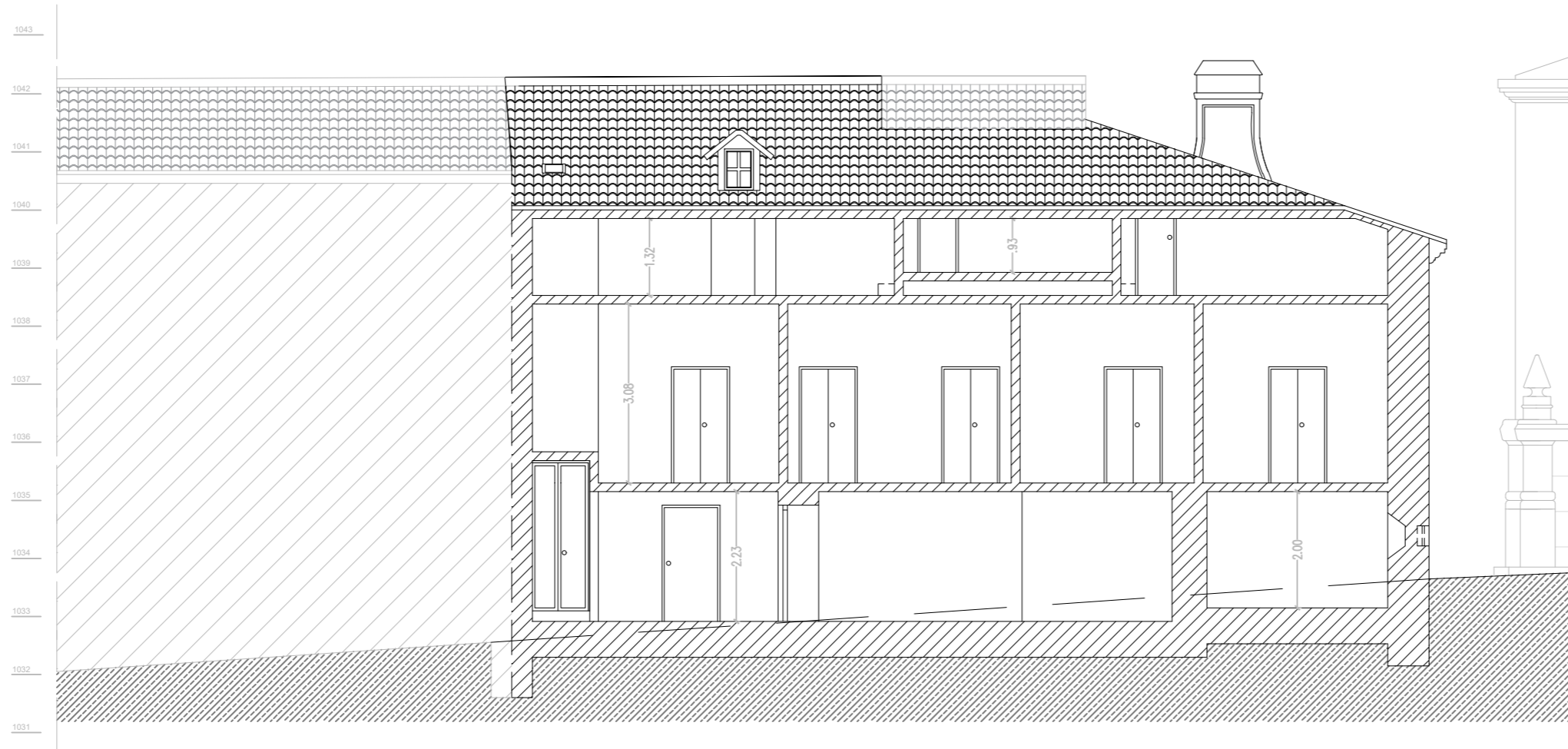
Corte E-F
