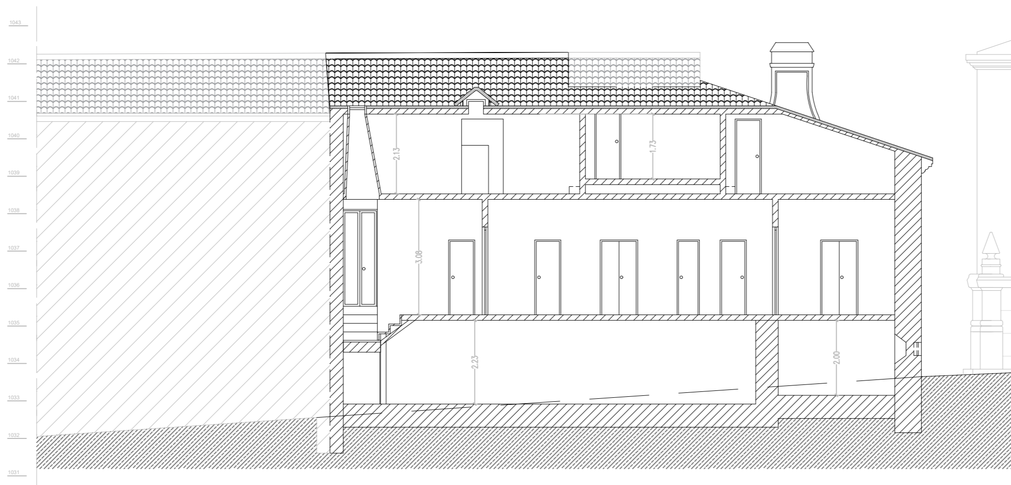
Corte G-H
