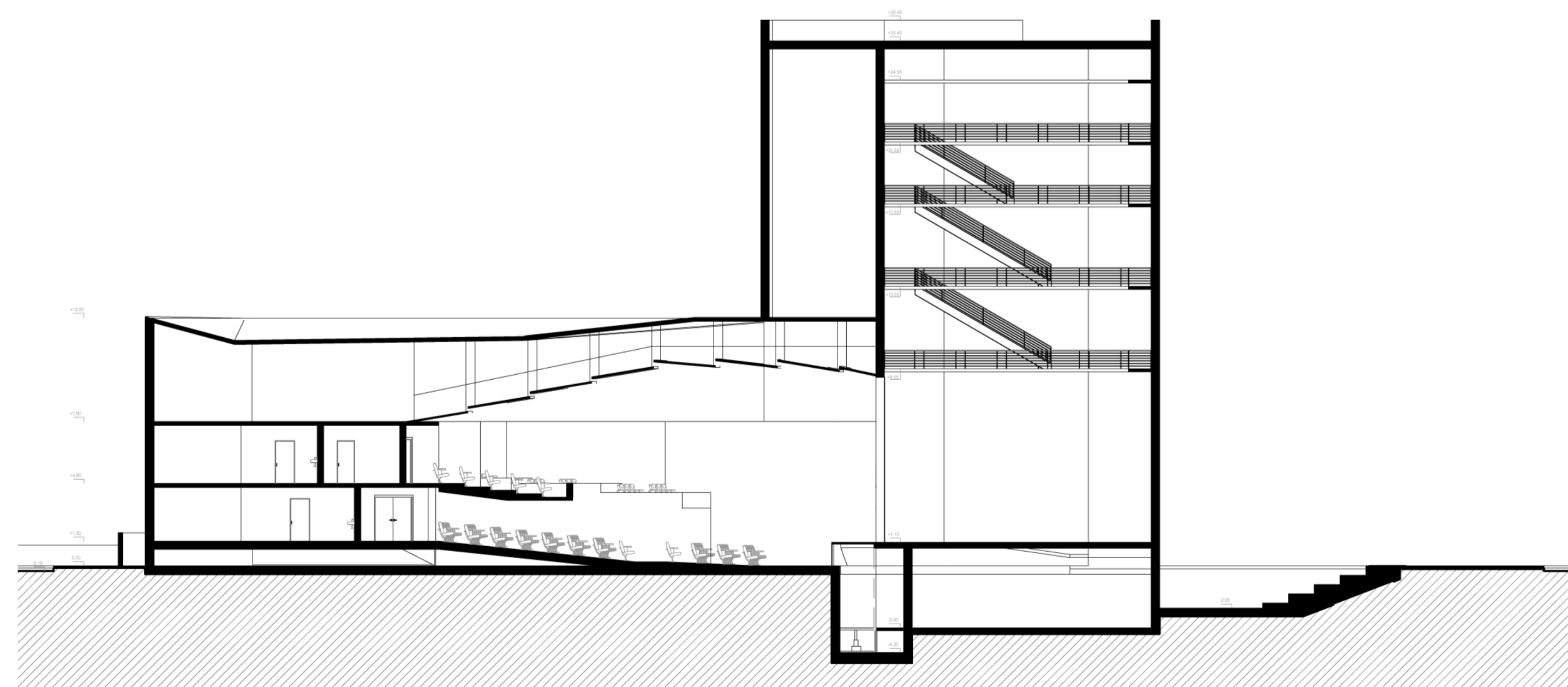
Corte Transversal
