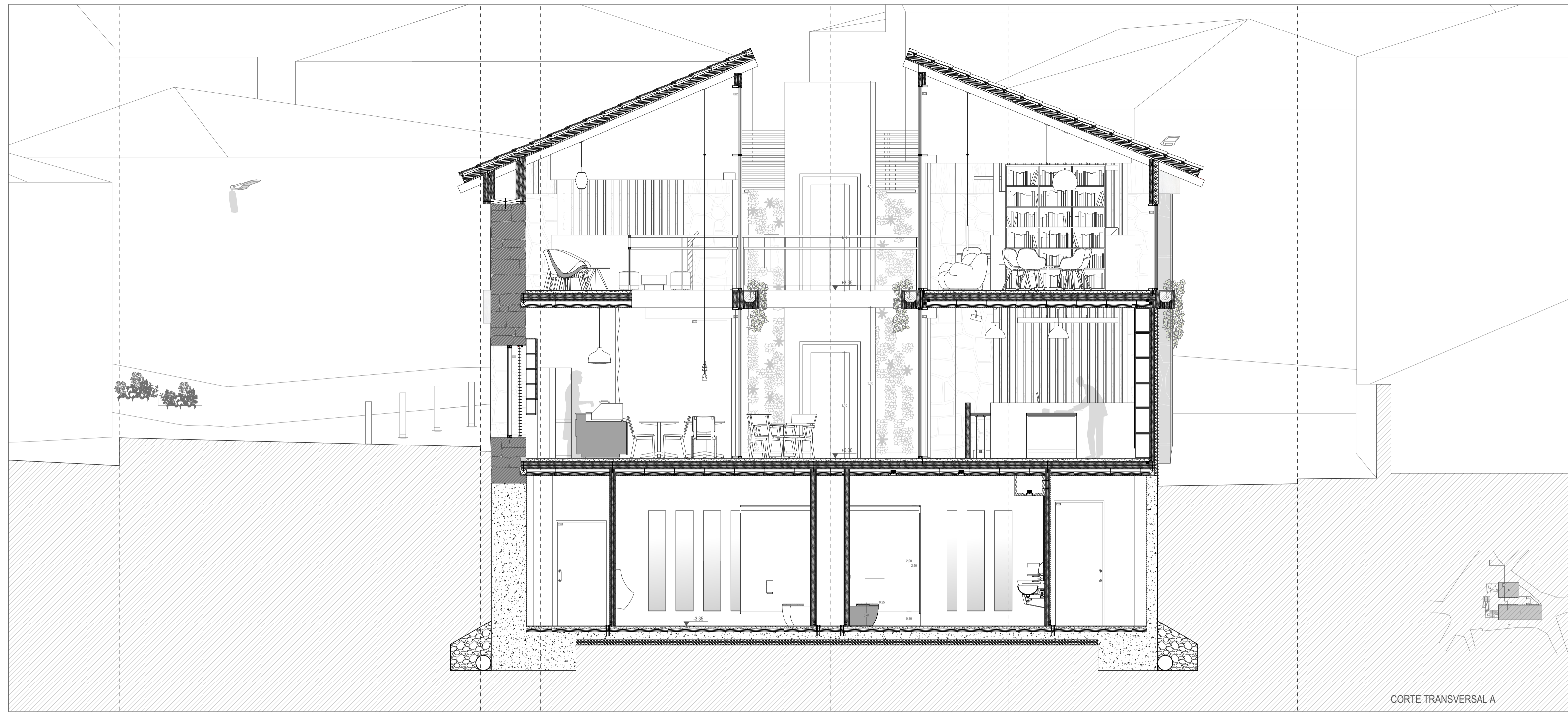
CORTE TRANSVERSAL A
