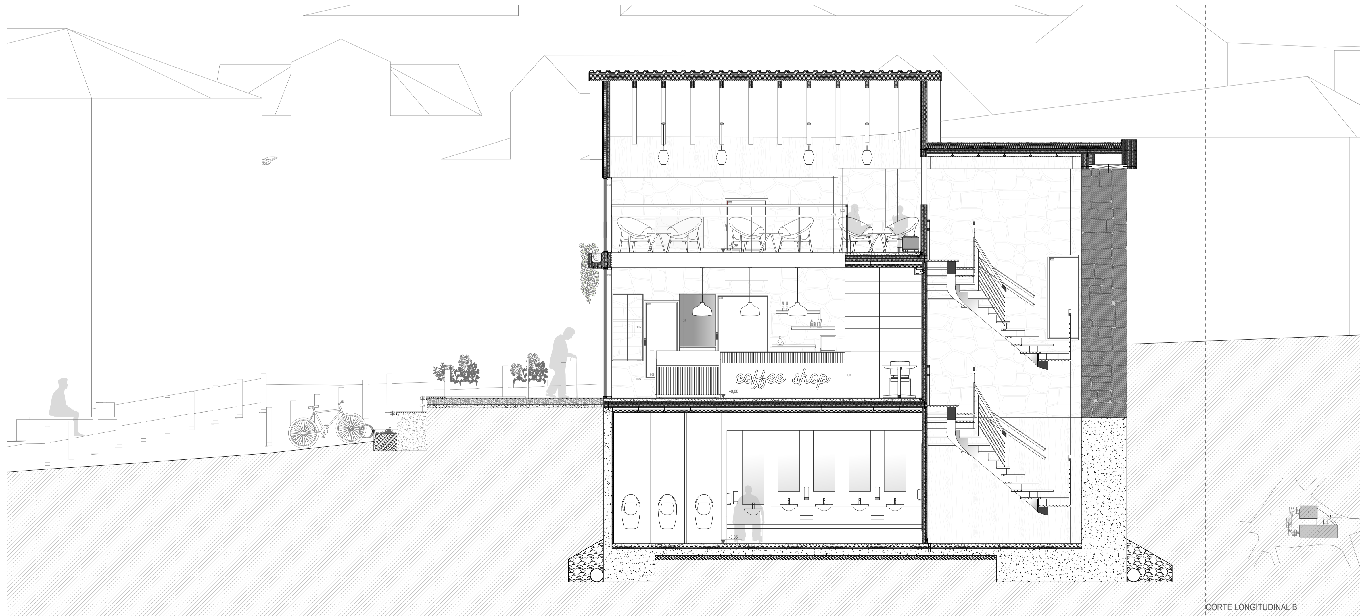
CORTE LONGITUDINAL B
