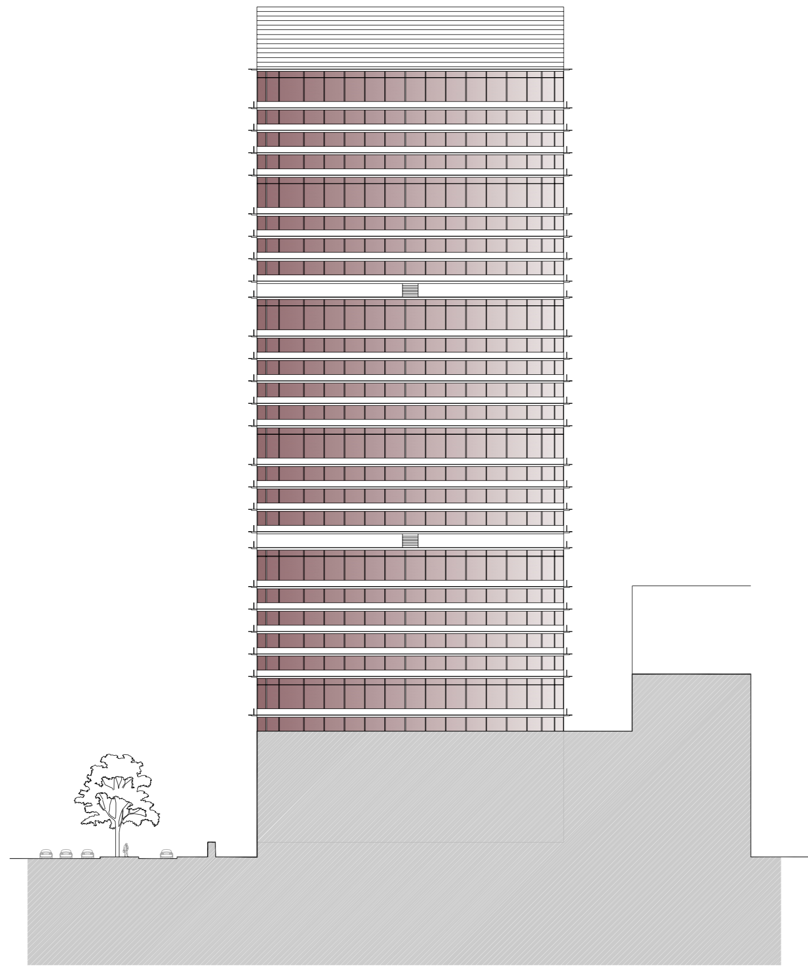
Alçado Norte
