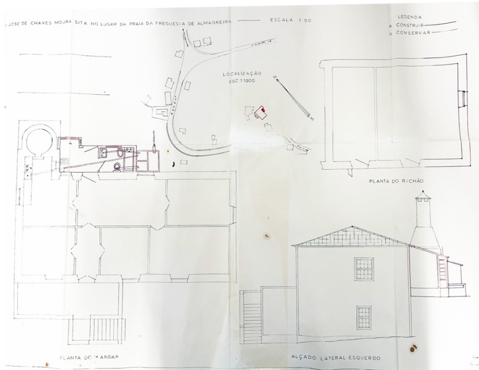
Figura 64 - Plantas e Alçado da casa balcão alongada, Praia Formosa
