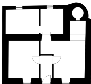
PLANTA DE PISO TÉRREO - 1:100
