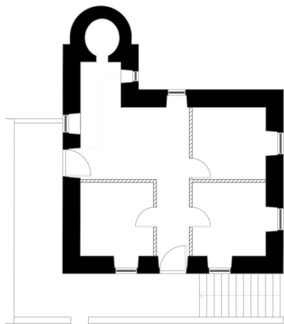
Planta de Piso Térreo
