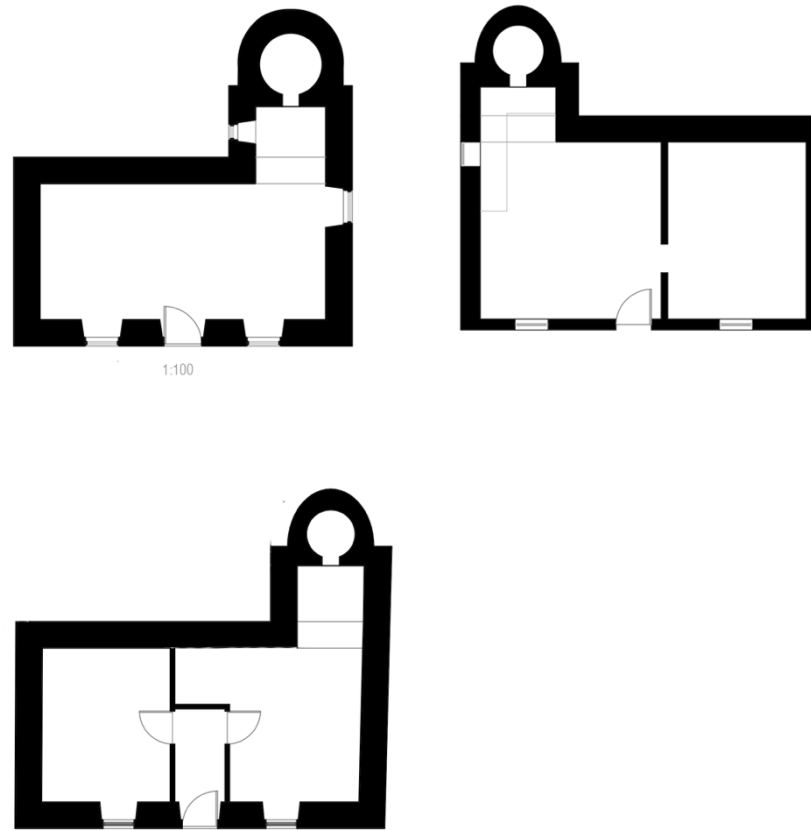
Figura 39 - Plantas de modelos de casa típica, 2023
