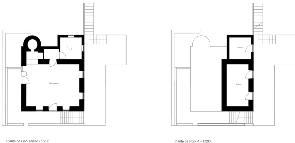
Figura 93 - Plantas de piso da casa balcão reabilitada, em Santa Bárbara, 2023
