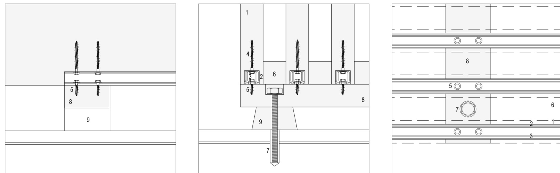
PORMENORA 1 painel de madeira de cerejeira 50 x 1493 x 2750mm 2 calha apolo 30 x 33 x 1393 x 2mm 3 calha U 22 x 22 x 1393 x 2mm 4 parafuso tirefond, inox A4 70 x 5 mm 5 parafuso tirefond, inox A4 30 x 5 mm 6 ripa de madeira de cerejeira 50 x 50 x 1801mm 7 ancoragem metálica com parafuso sextavado 12 x 150 mm 8 caibro de madeira de cerejeira 100 x 100 x 4450 mm 9 apoio do barrote de madeira de cerejeira 50 x 100 x 100mm
