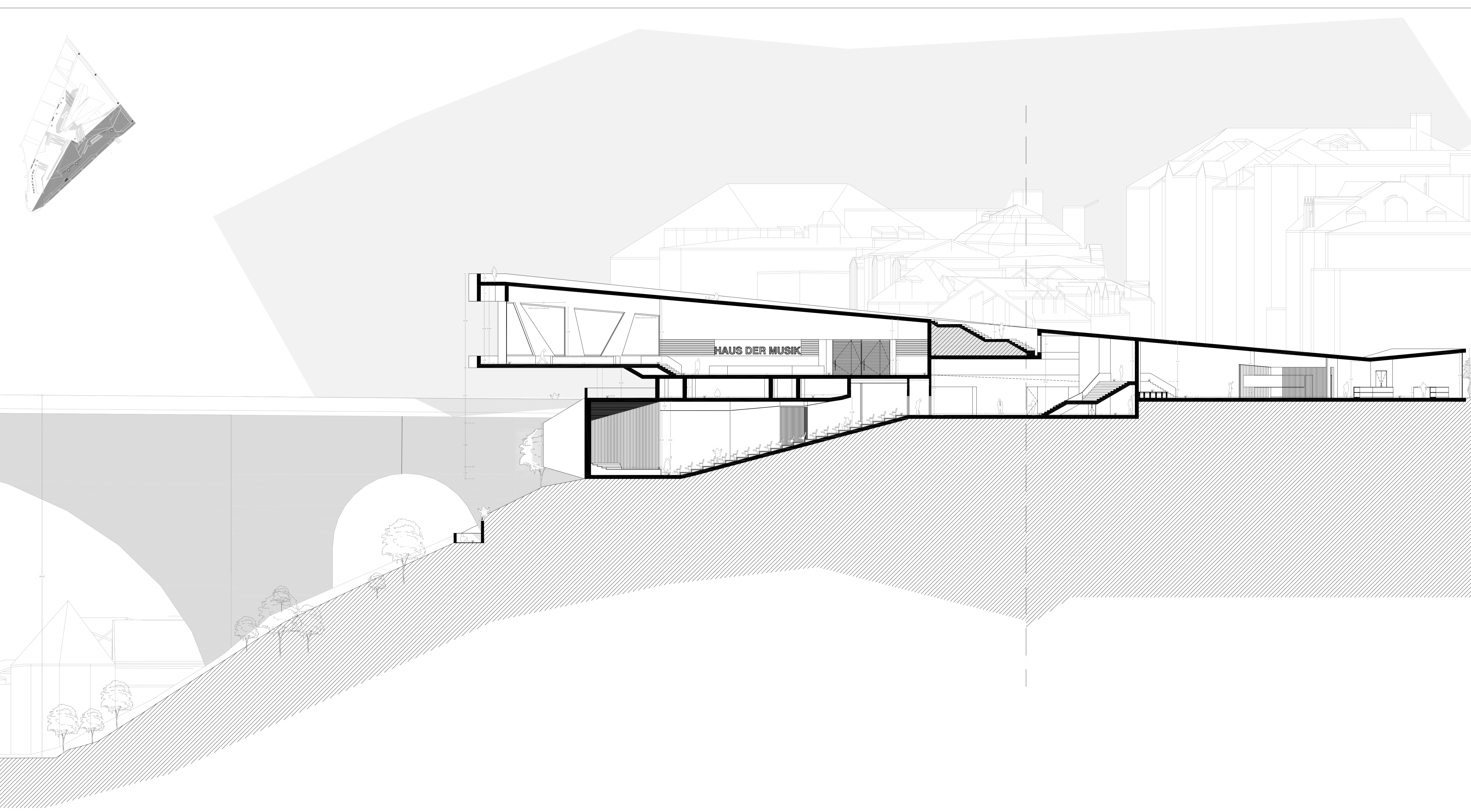
corte | C-C'
