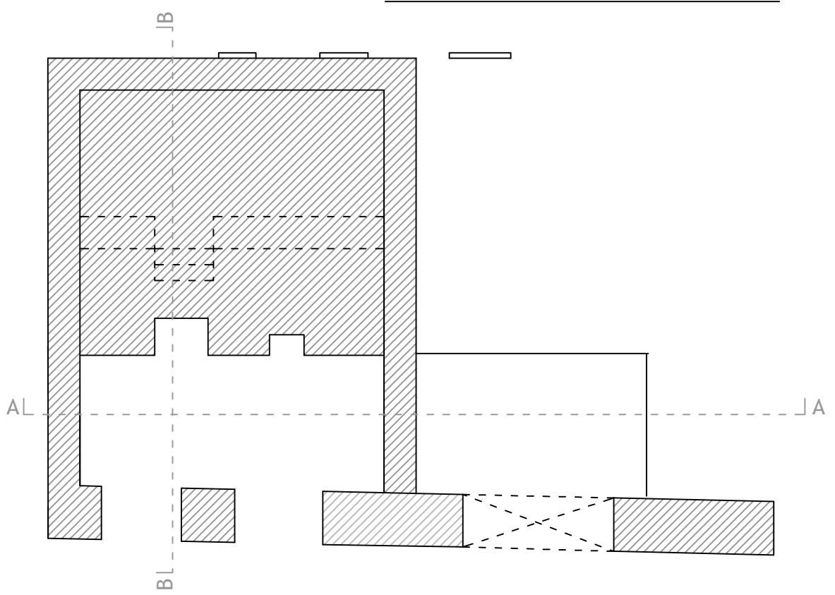
Planta -1
