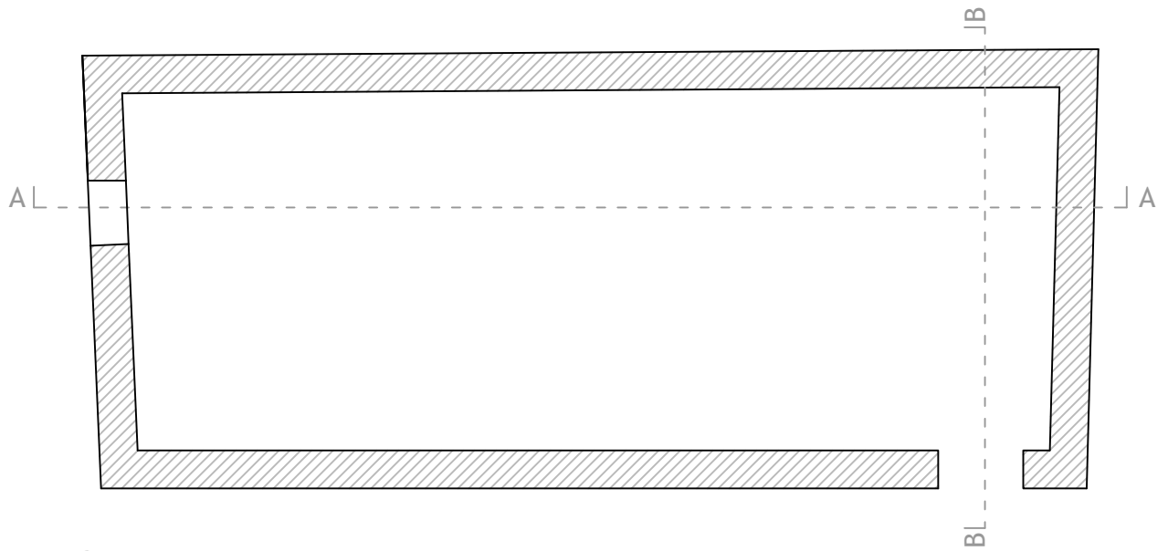
Planta | Escala 1:100
