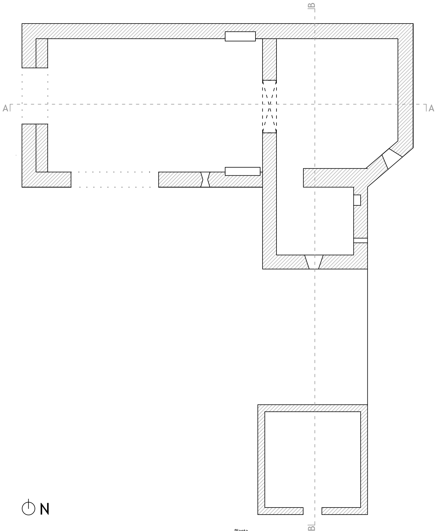
Planta
