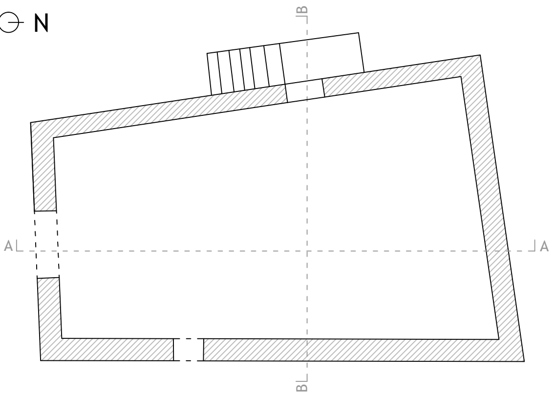
Planta
