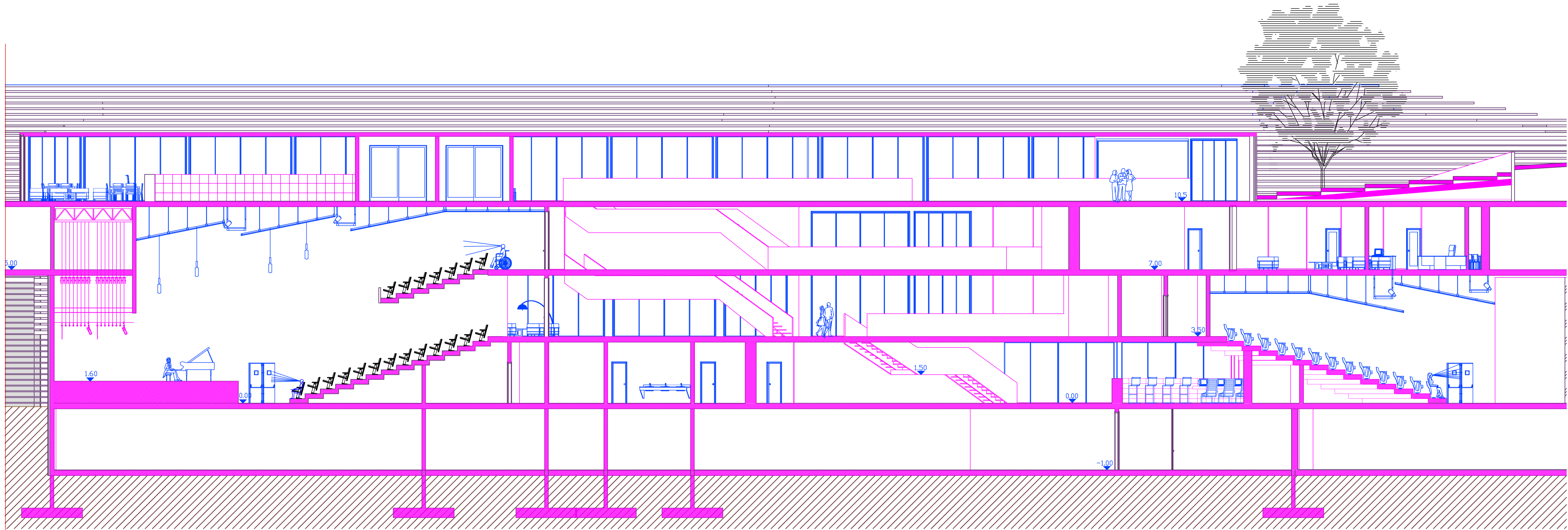
corte 9
