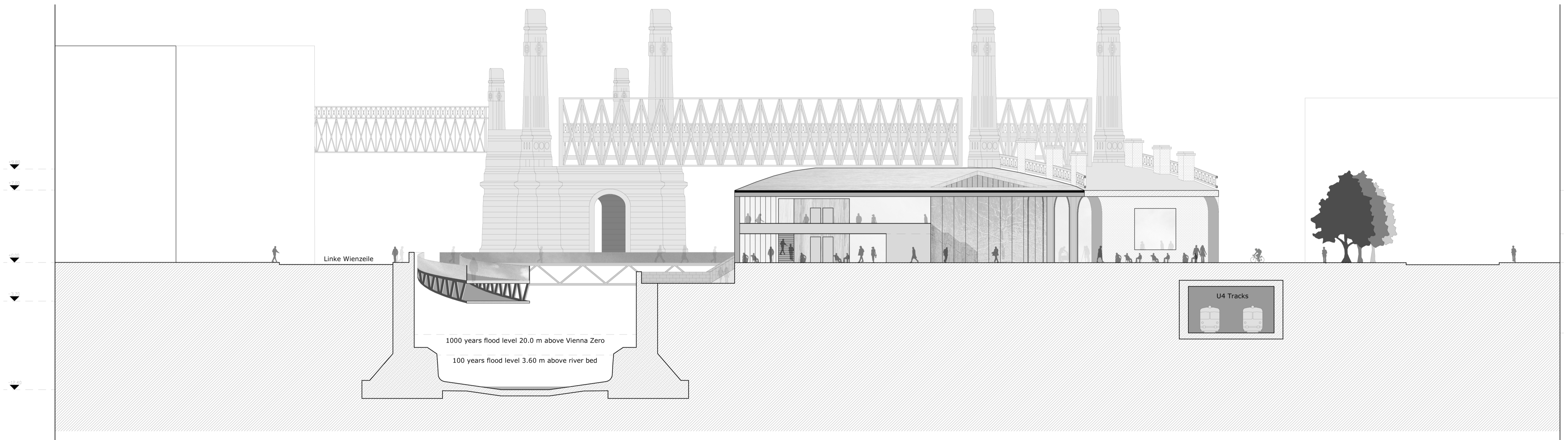
Corte C2
