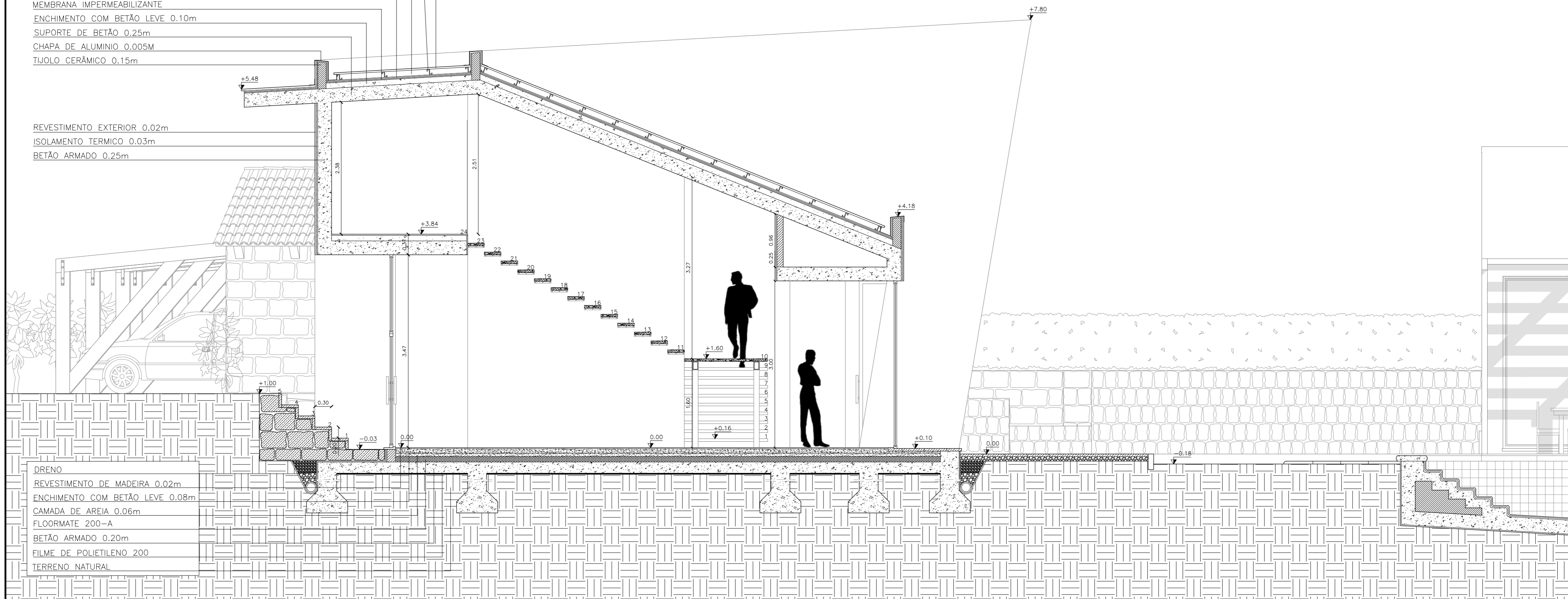
CORTE A/A' ESCALA 1:50
