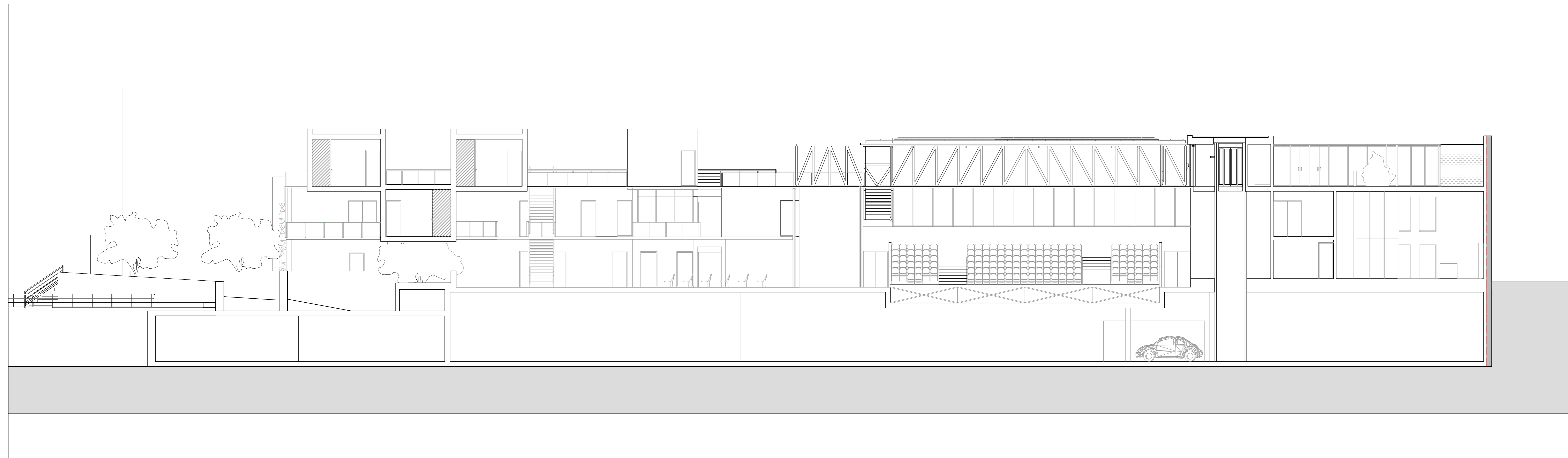
PERFIL LONGITUDINAL 1
