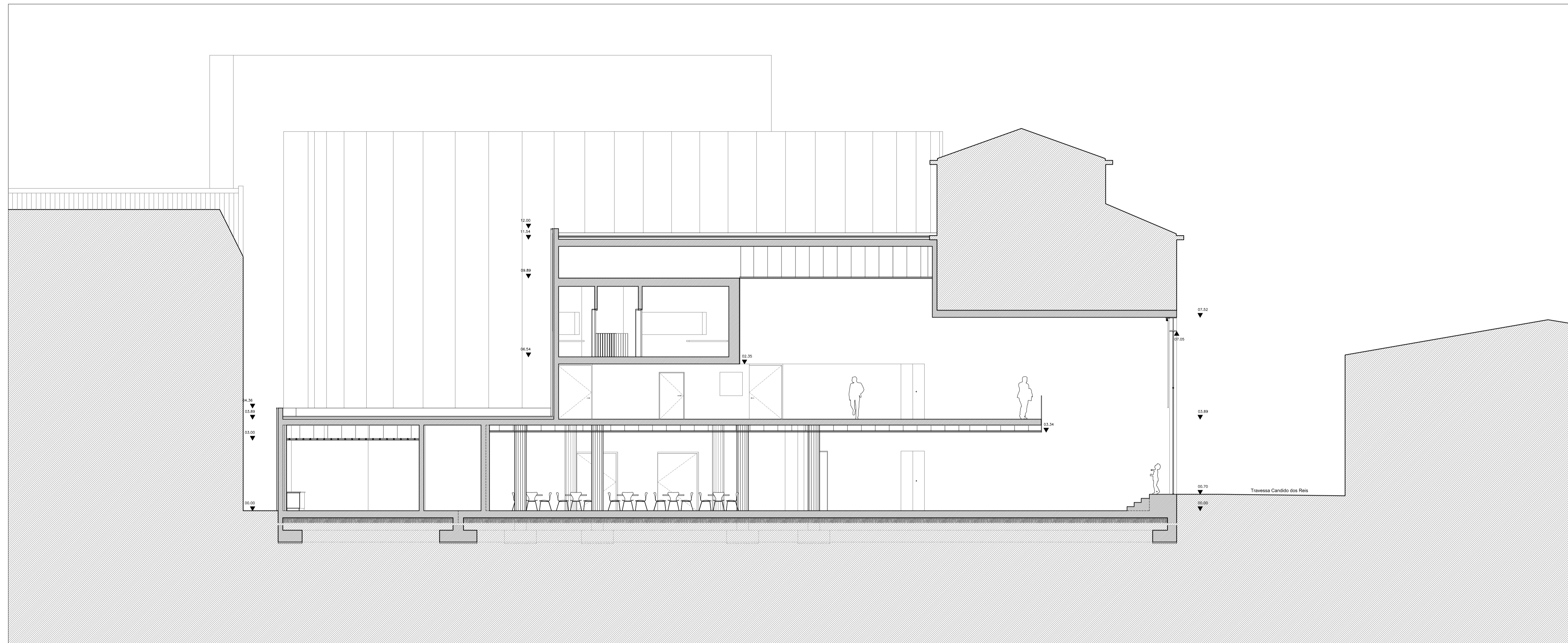
CORTE TRANSVERSAL - CT02
