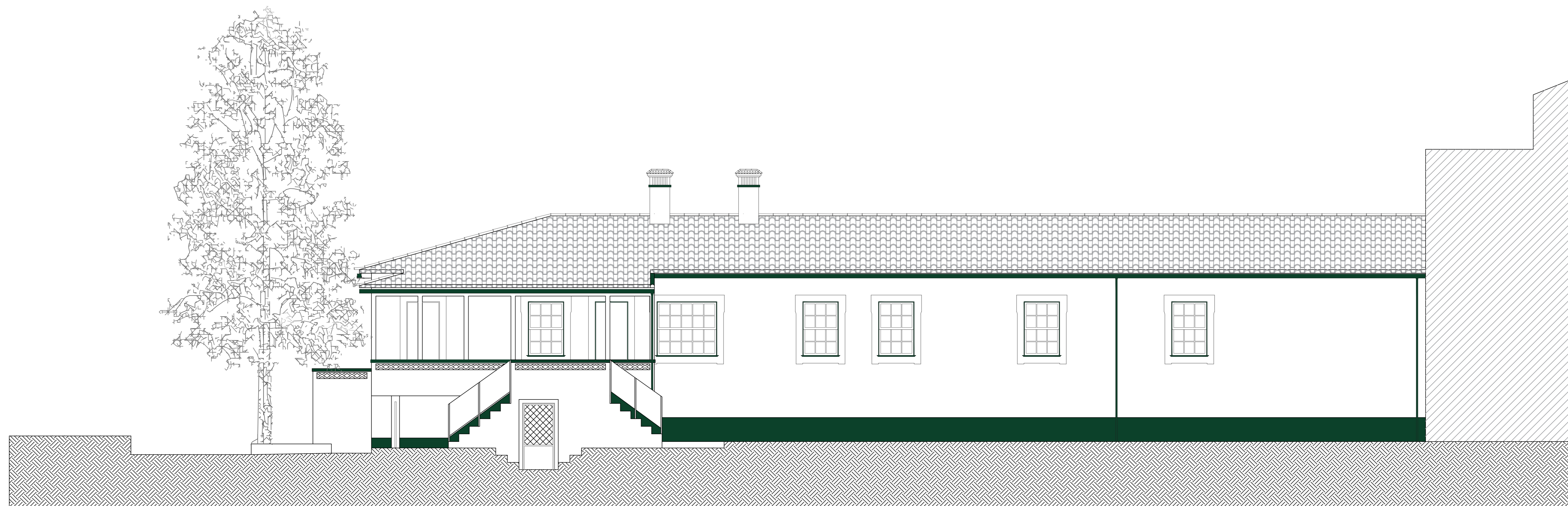
Alçado Posterior
