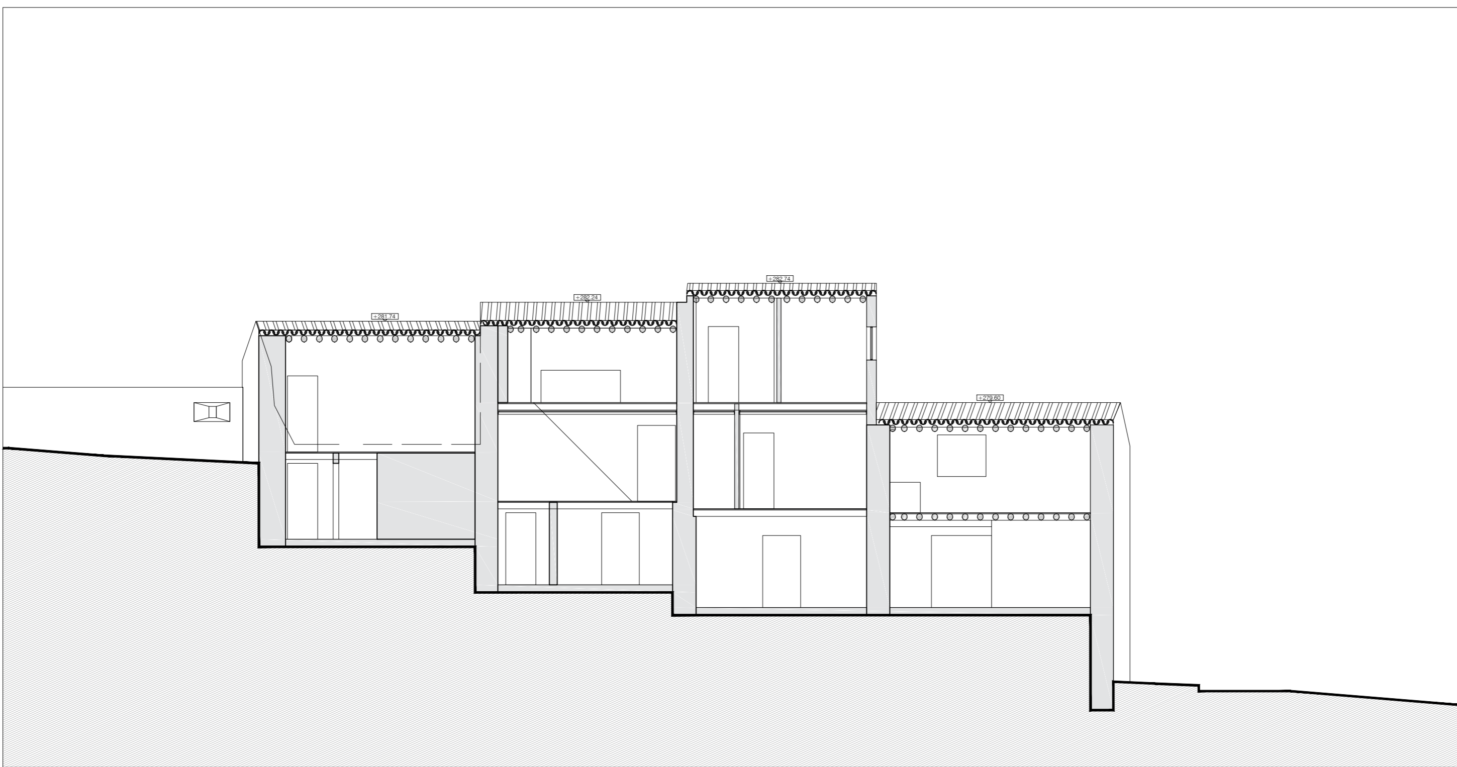
ALÇADO 03 ANEXOS CASA PINA FALCÃO
