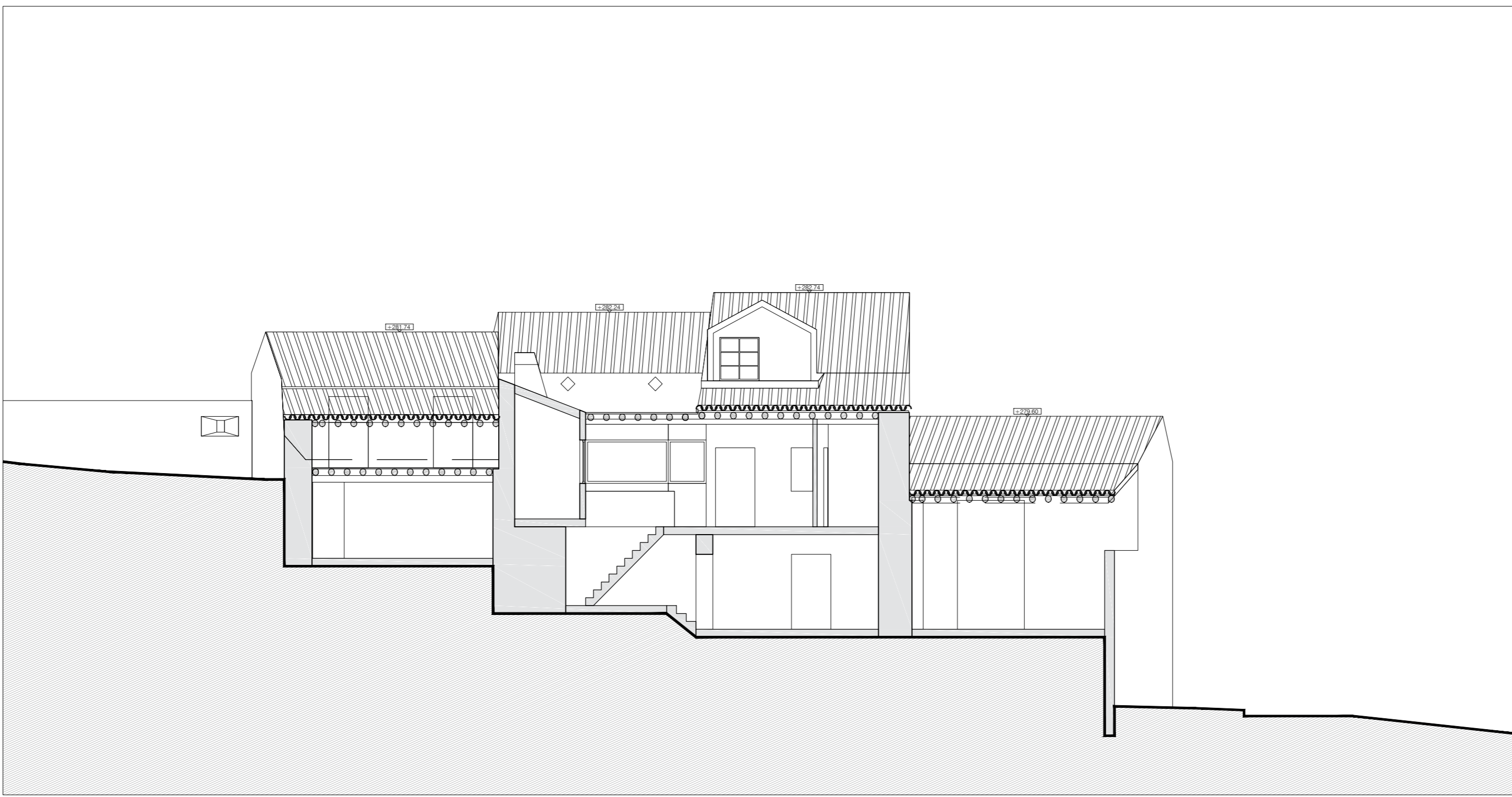
CORTE 02 ANEXO CASA PINA FALCÃO
