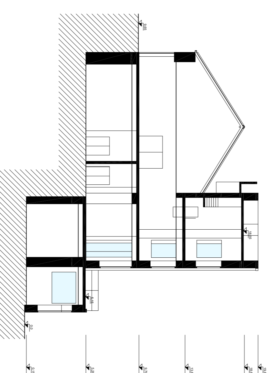
Corte CC'
