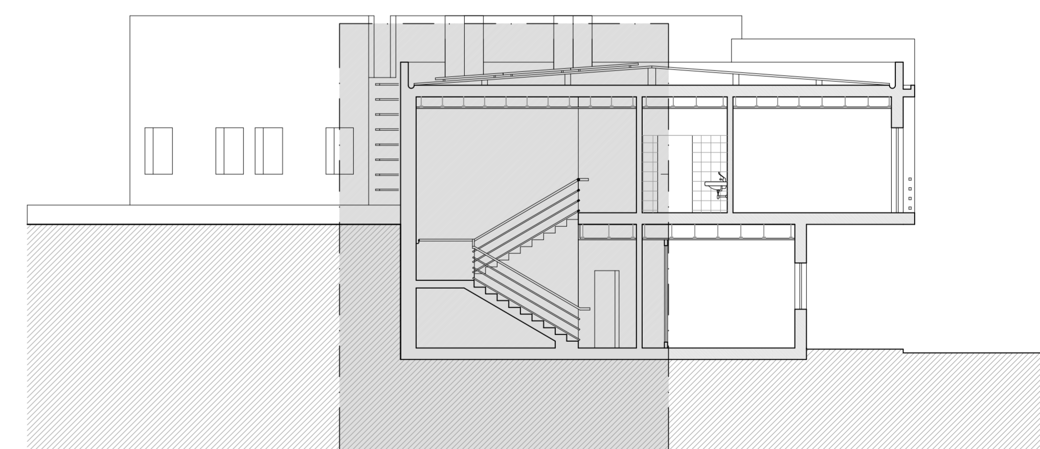
CORTE C-C PROPOSTO
