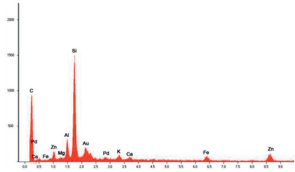
Fig. 14. Análise do espectro da figura 13 com o pormenor de um possível resto de escória de fundição.
