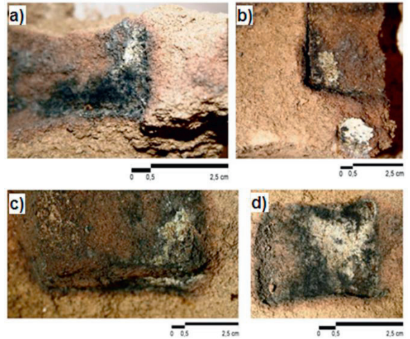
Fig. 10. Detalhe da zona de interface entre o bronze e o árido da Panasqueira: a) e b) pormenores da mistura de 15%, c) e d) pormenores da mistura de 25%.
