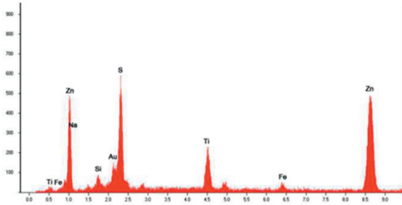
Fig. 12. Análise do espectro da figura 11 com elevada presença de enxofre, zinco e titânio (possivelmente do agregado) e sódio (possivelmente proveniente da paragonite ou da albite, minerais presentes no agregado).
