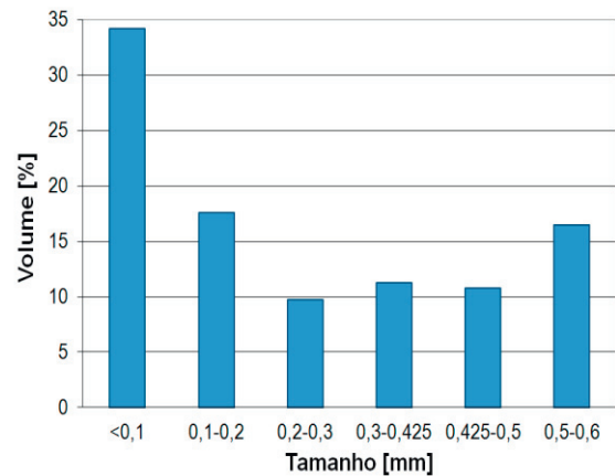
Fig. 5. Análise granulométrica do agregado fino da Panasqueira moído.
