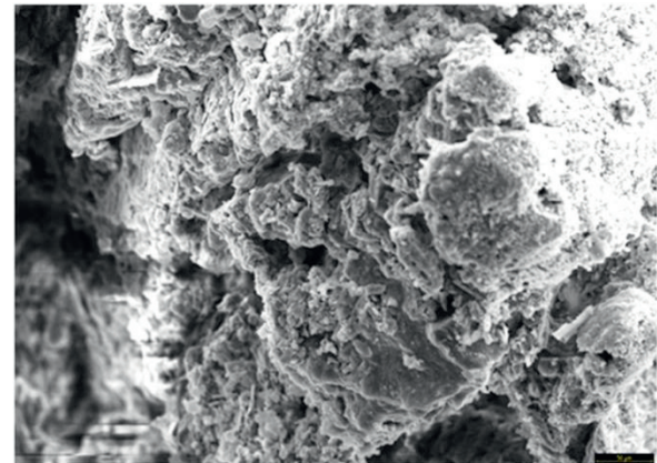
Fig. 16. Micrografia (SEM) com ampliação de 200 vezes da região de difusão térmica da mistura refratária de 25%.
