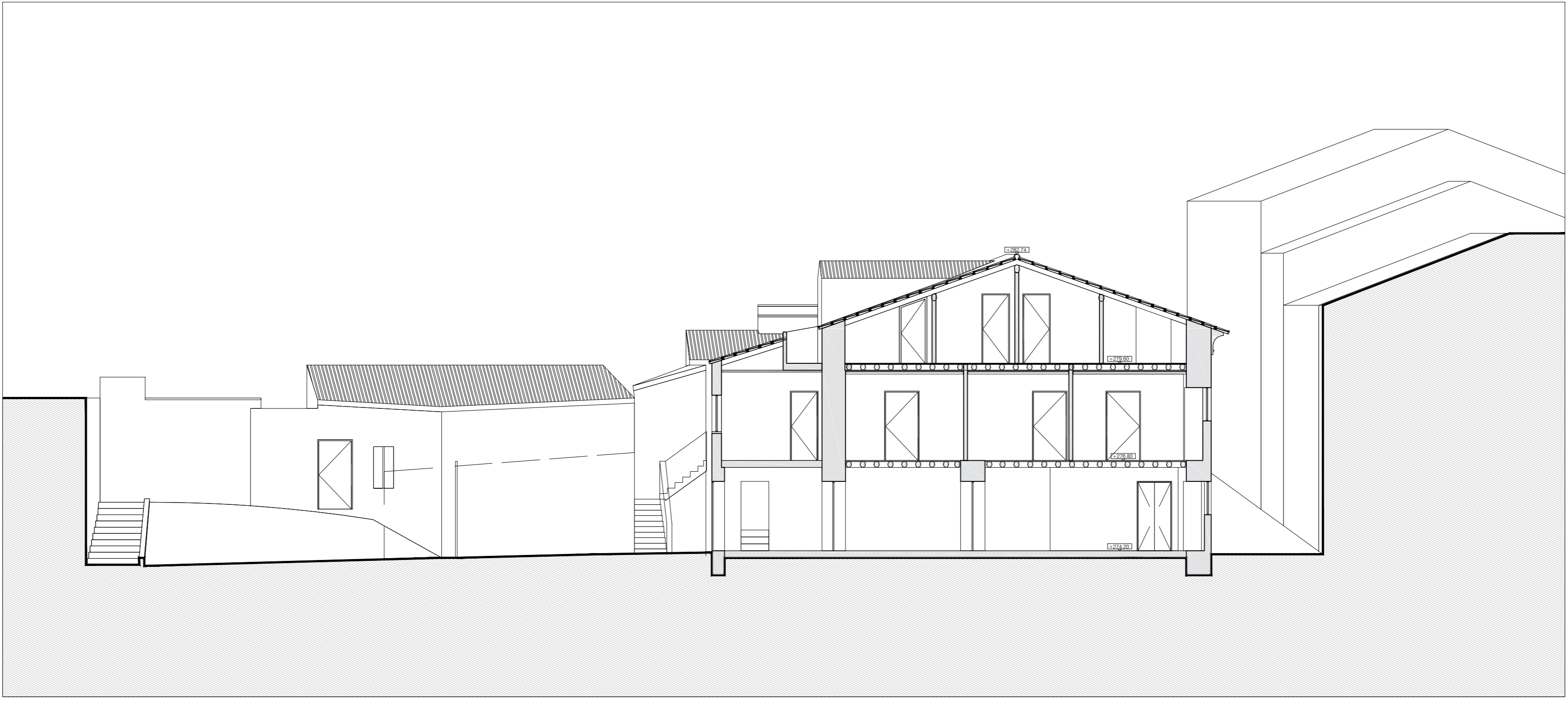
CORTE S2 ANEXO CASA PINA FALCÃO
