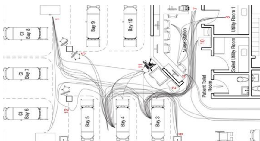
Figura 8 - Diagrama de esparguete. Fonte: http://www.array-architects.com/Lean-applied-to-designing-a-dialysis-unit
