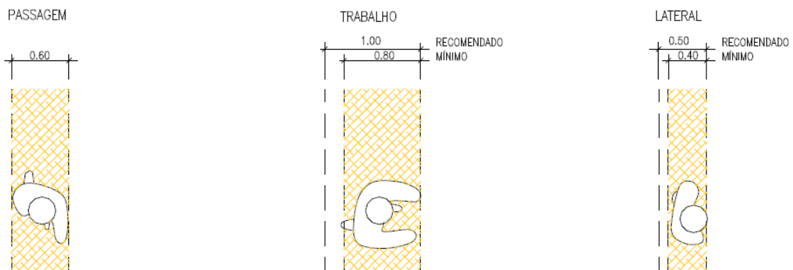
Figura 36 - Áreas recomendadas e mínimas em zonas de passagem frontal, lateral e de trabalho. Fonte: Paiva C., 2002, p. 23
