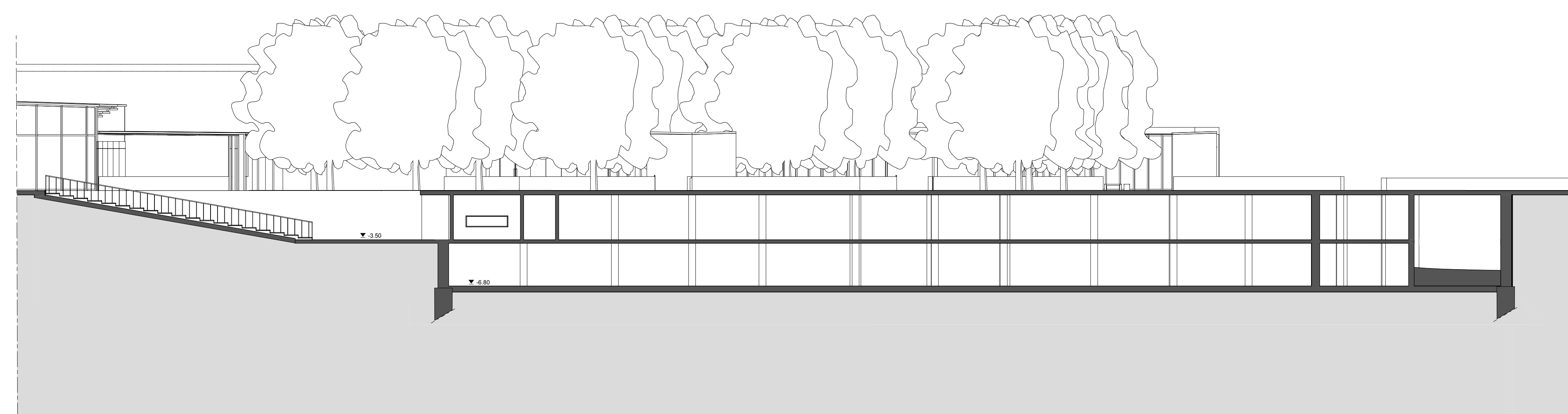
Corte 7
