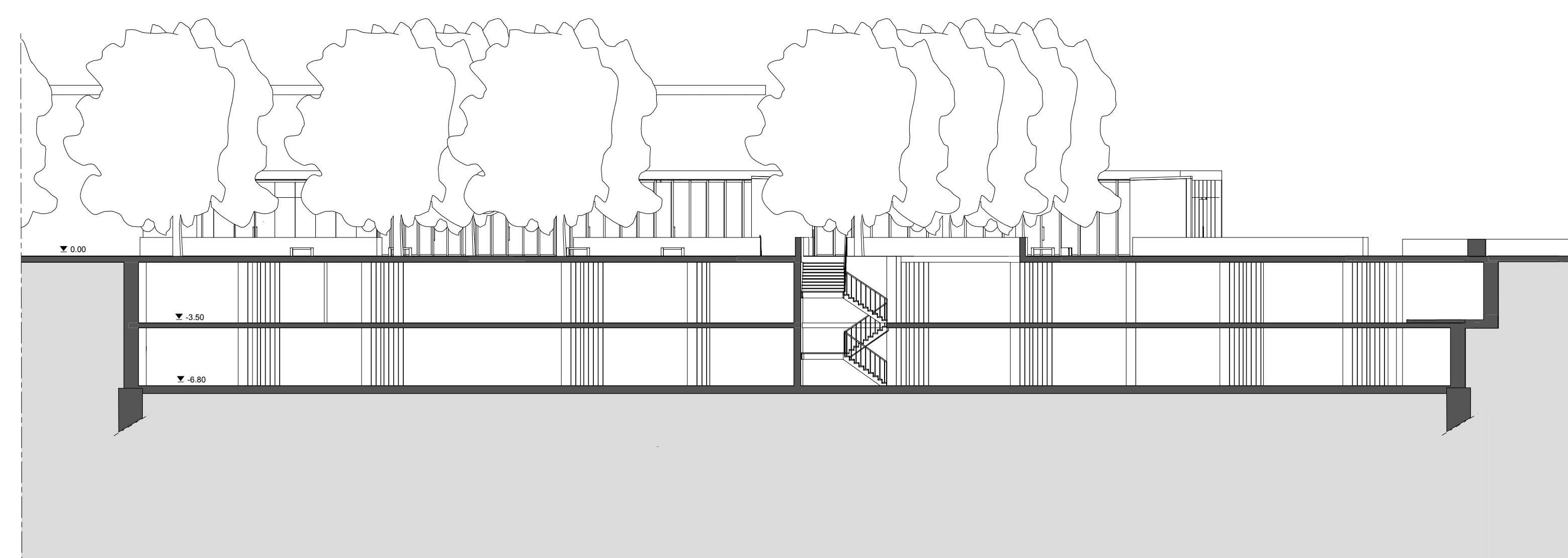
Corte 8
