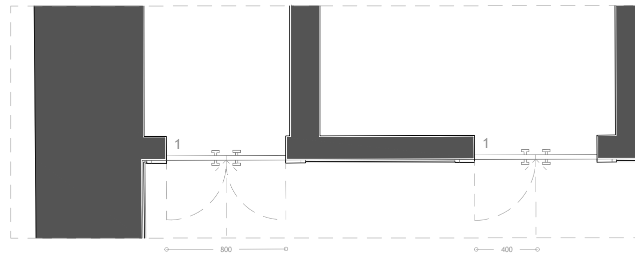
Imagem 173 - Levantamento gráfico da Porta P3 - Planta - Escala 1:25
