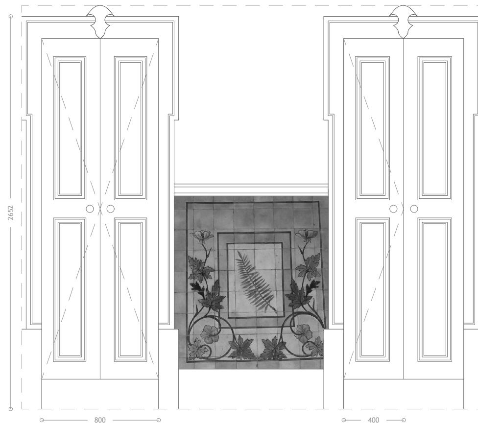
Imagem 171 - Levantamento gráfico da Porta P3 - Frente - Escala 1:25
