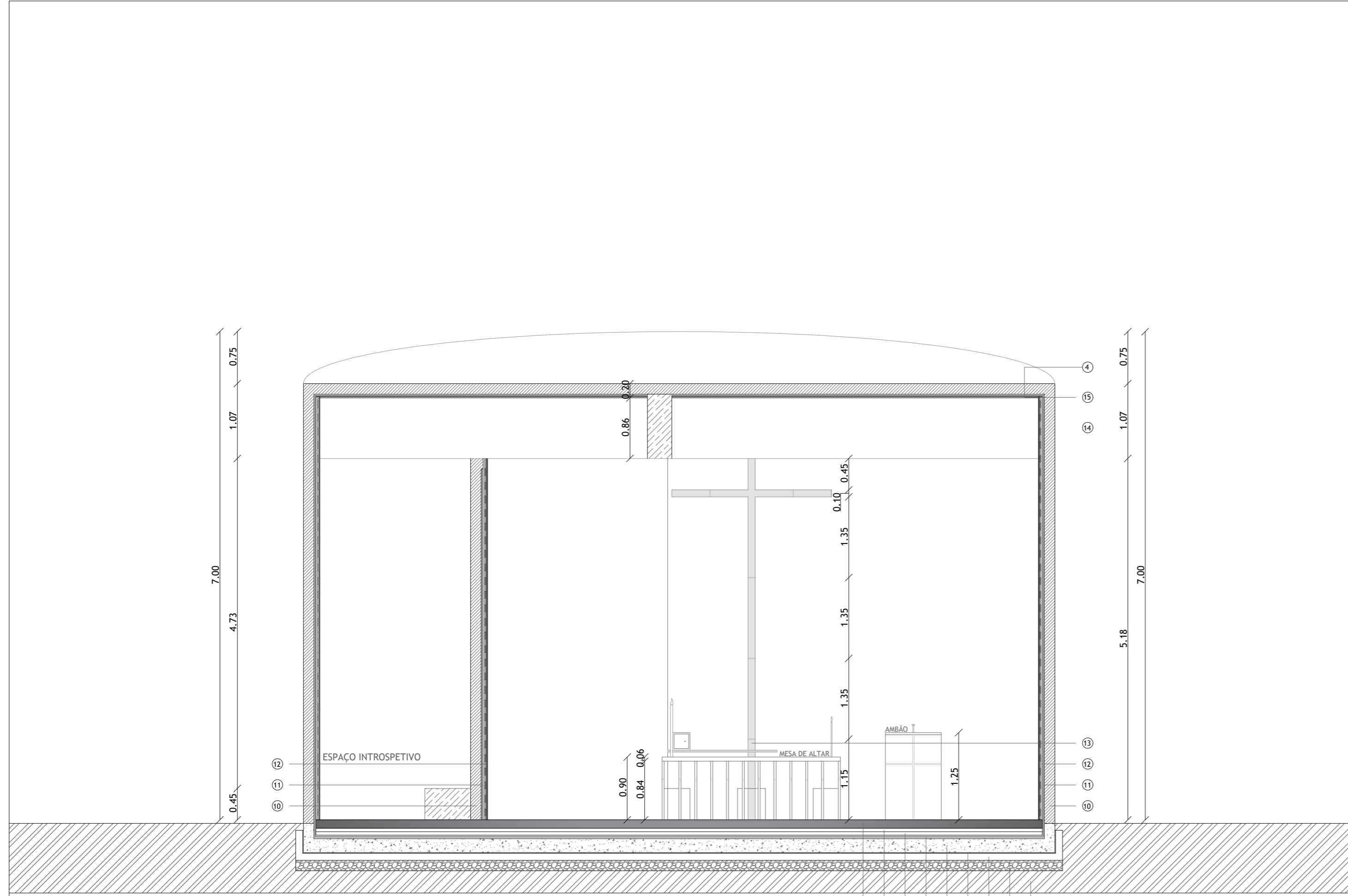
CORTE CC'
