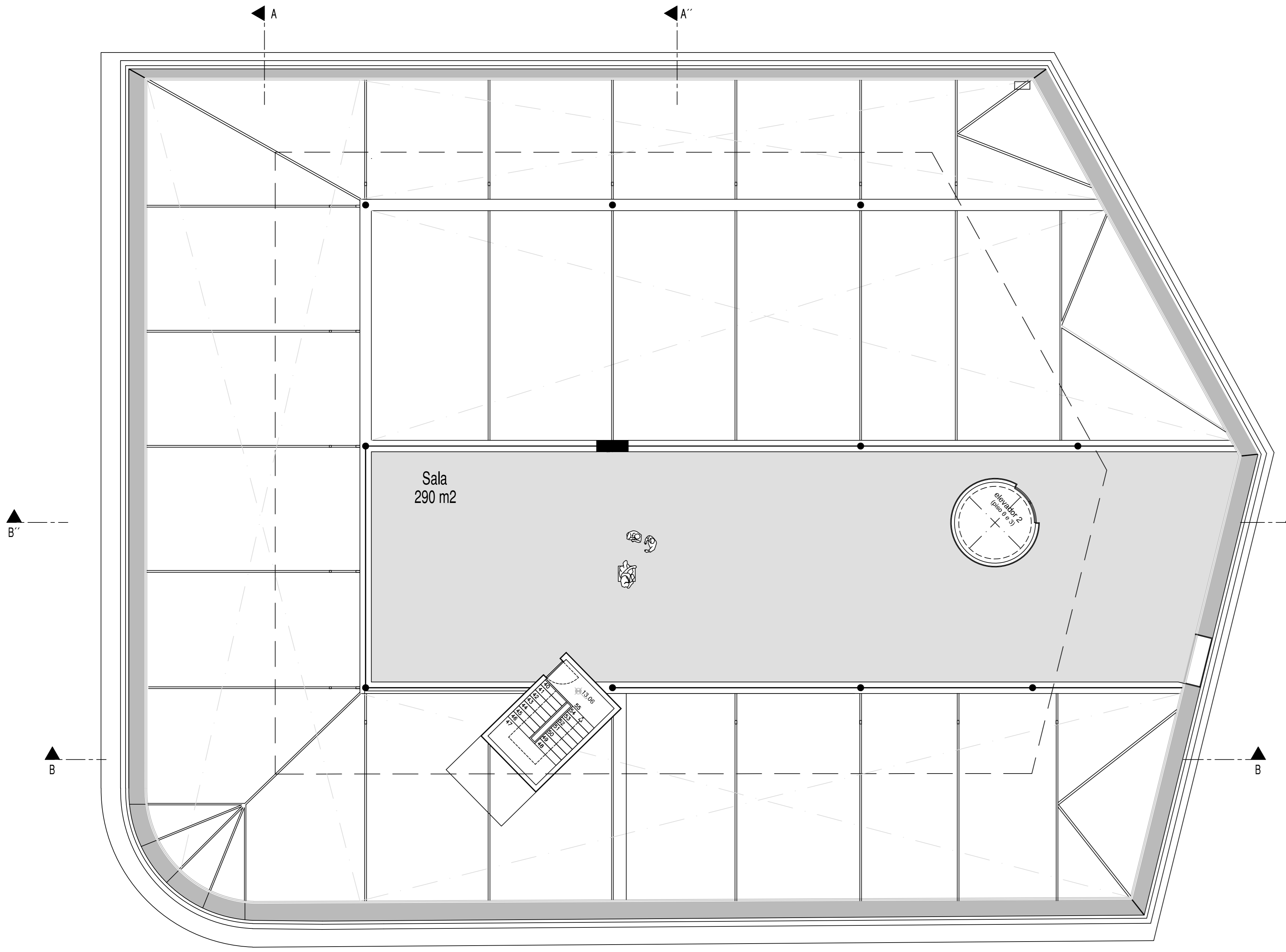
PISO 3
