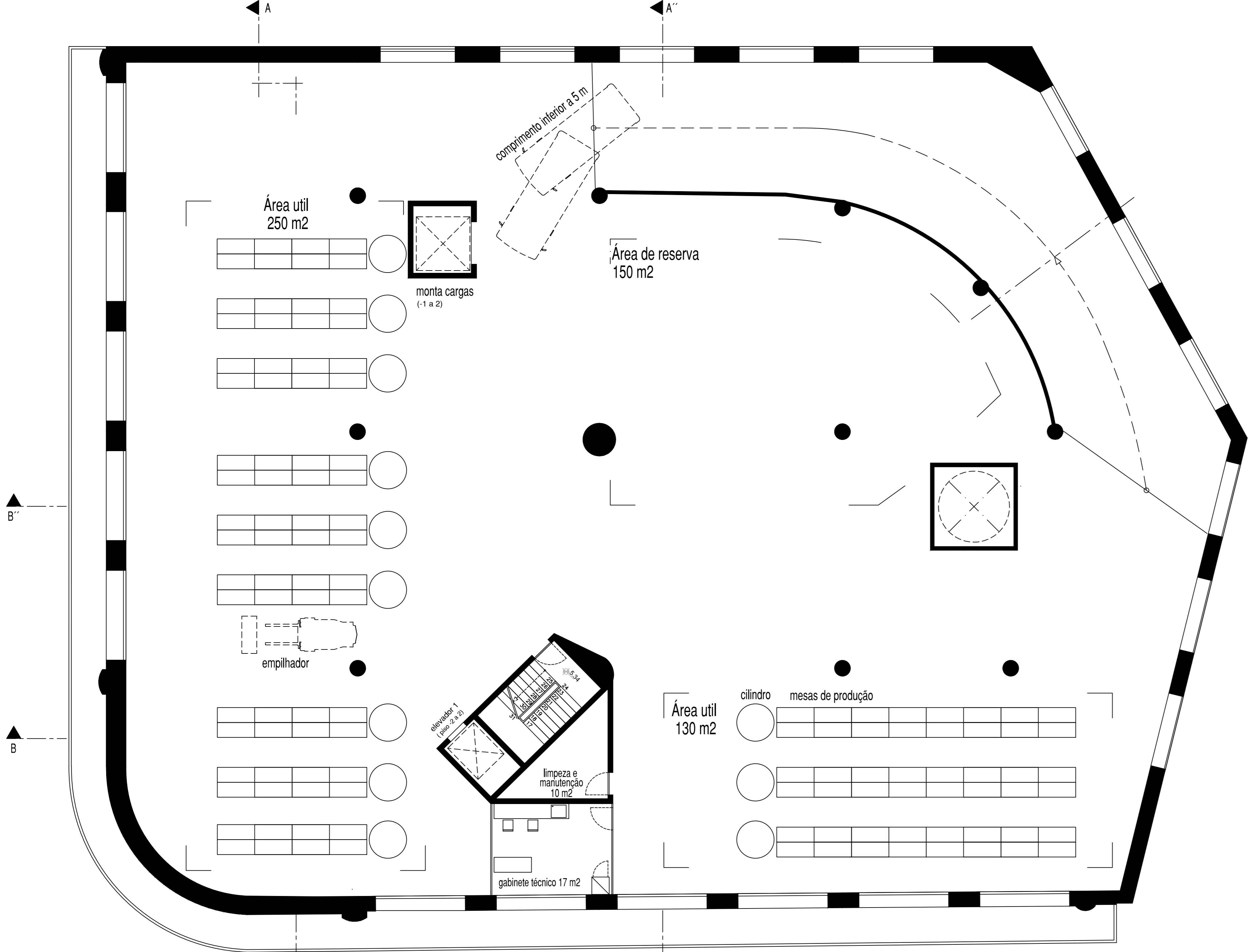
PISO 1
