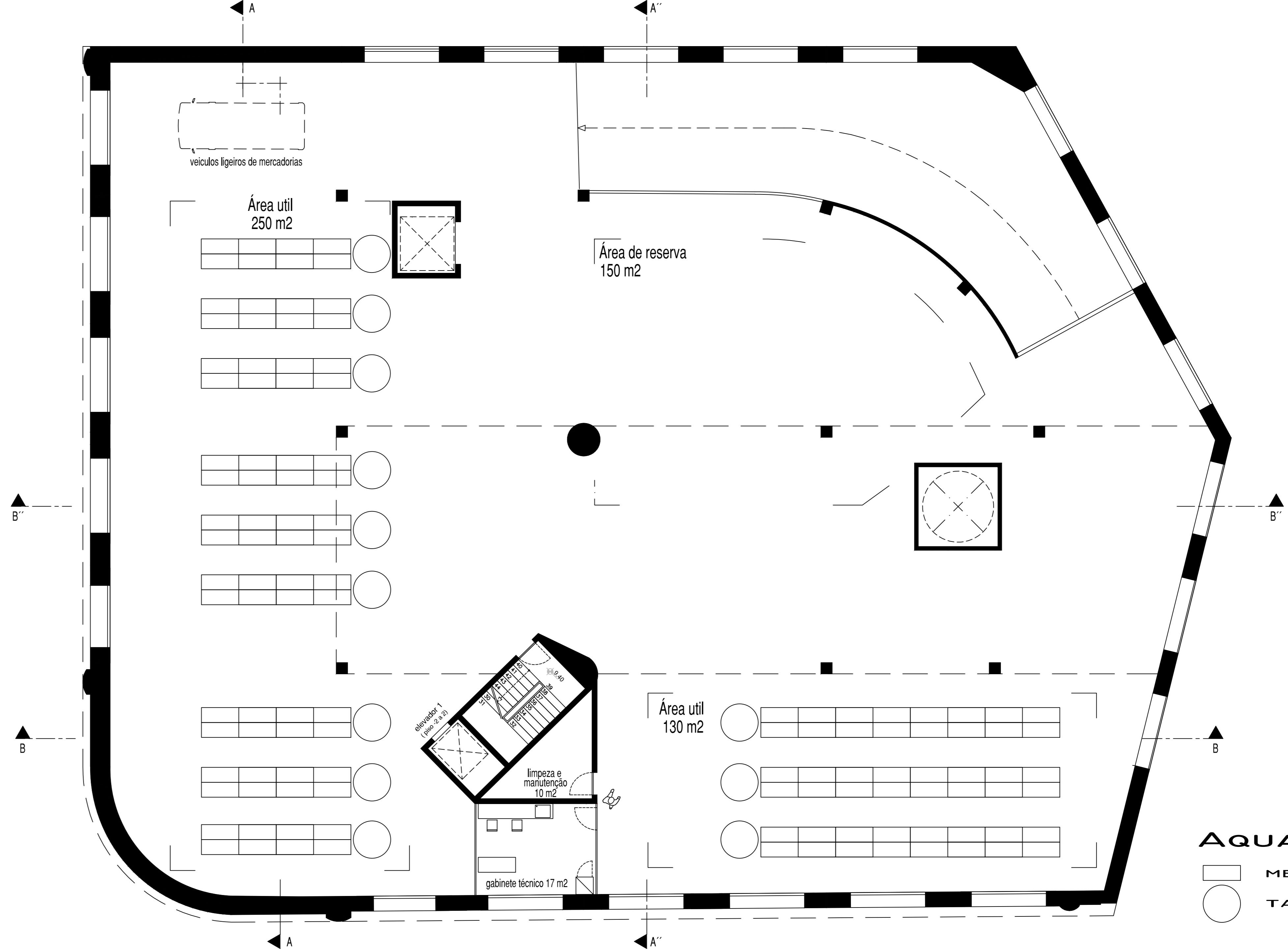
PISO 2
