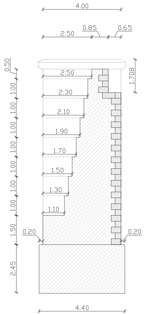
CORTE LONGITUDINAL DO ENCONTRO 1
