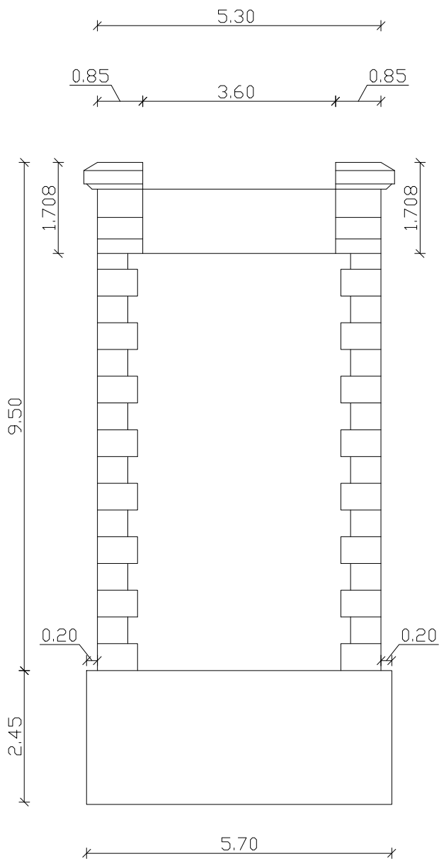
ALÇADO DO ENCONTRO 1
