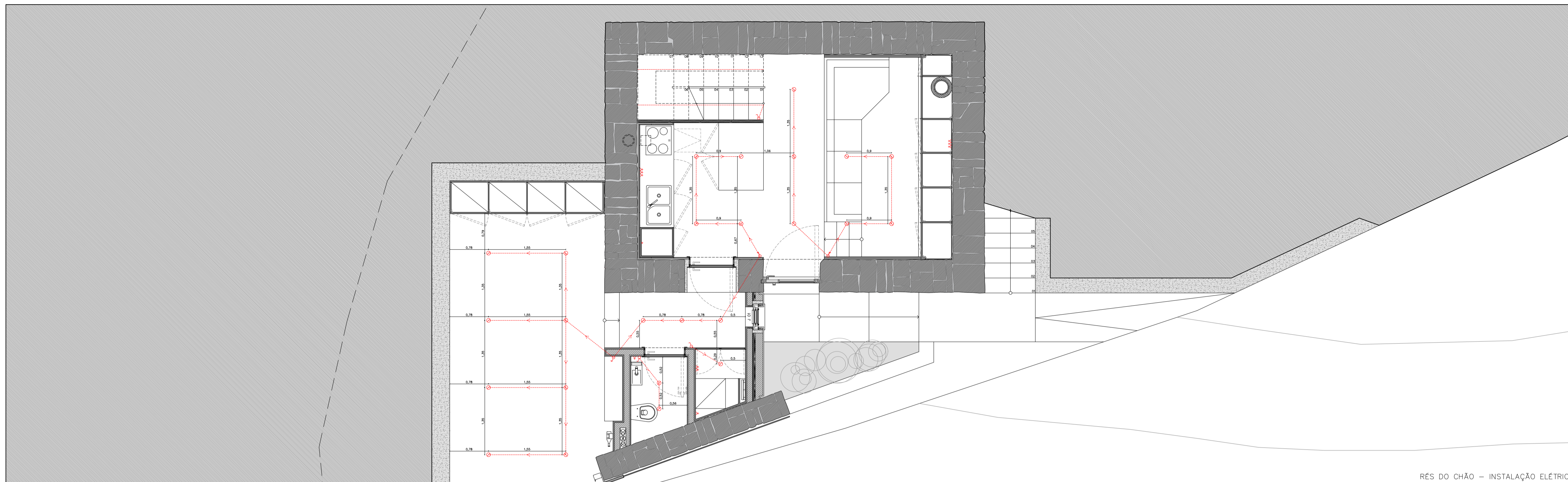
PISO DO CHÃO - INSTALAÇÃO ELÉTRICA
