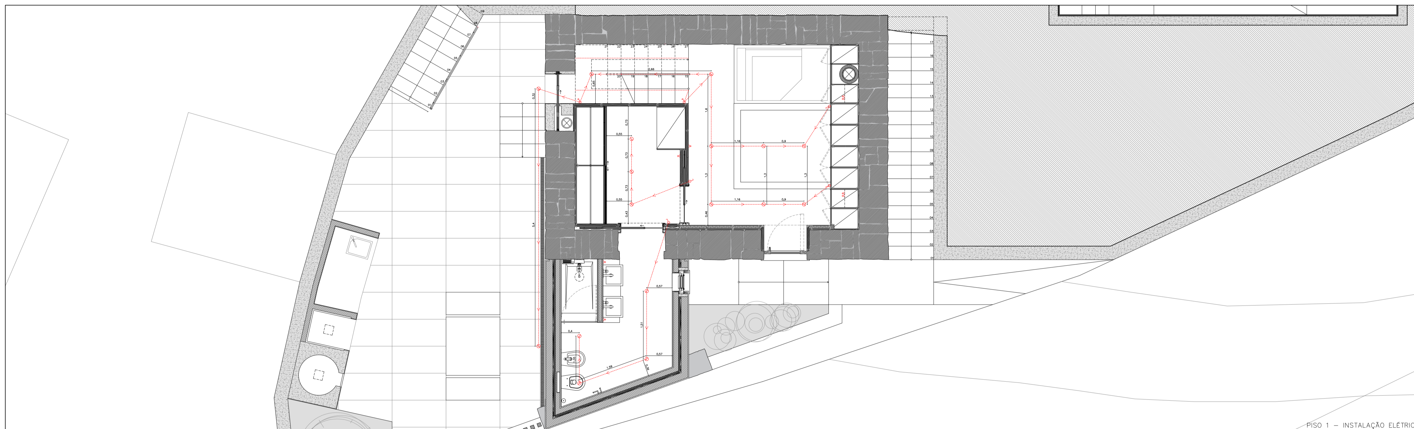
PISO 1 - INSTALAÇÃO ELÉTRICA
