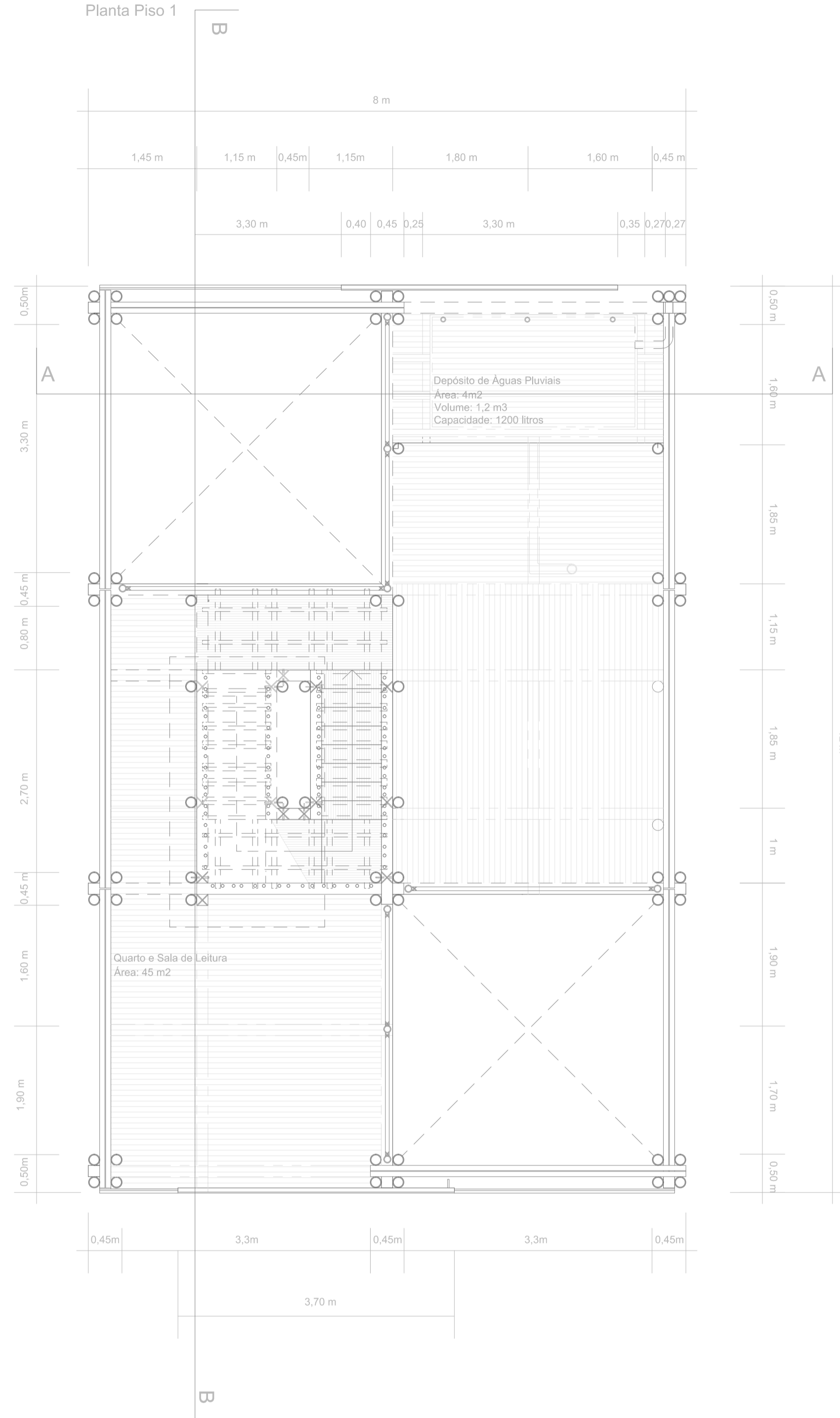
Planta Piso 1
