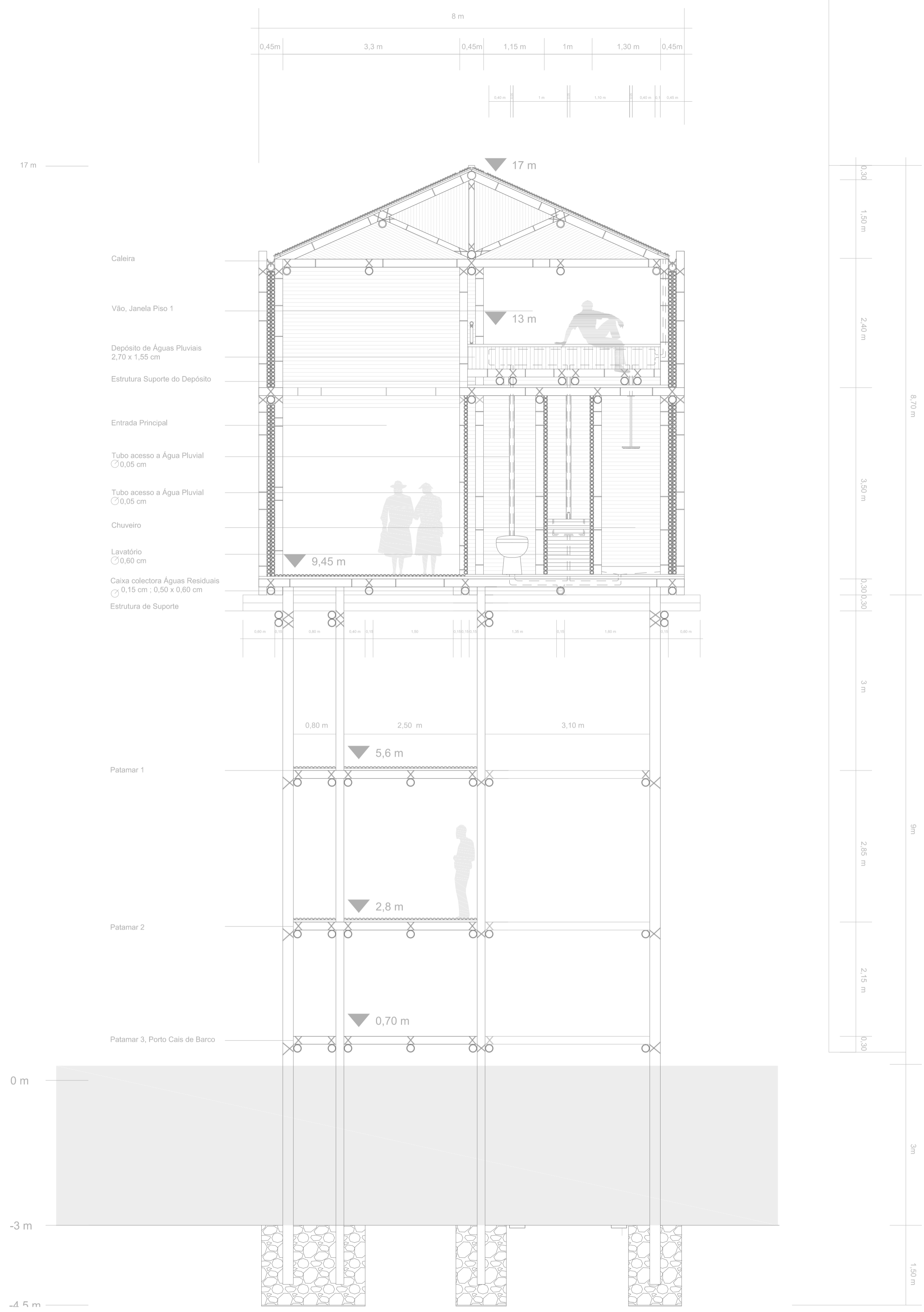
Corte A
