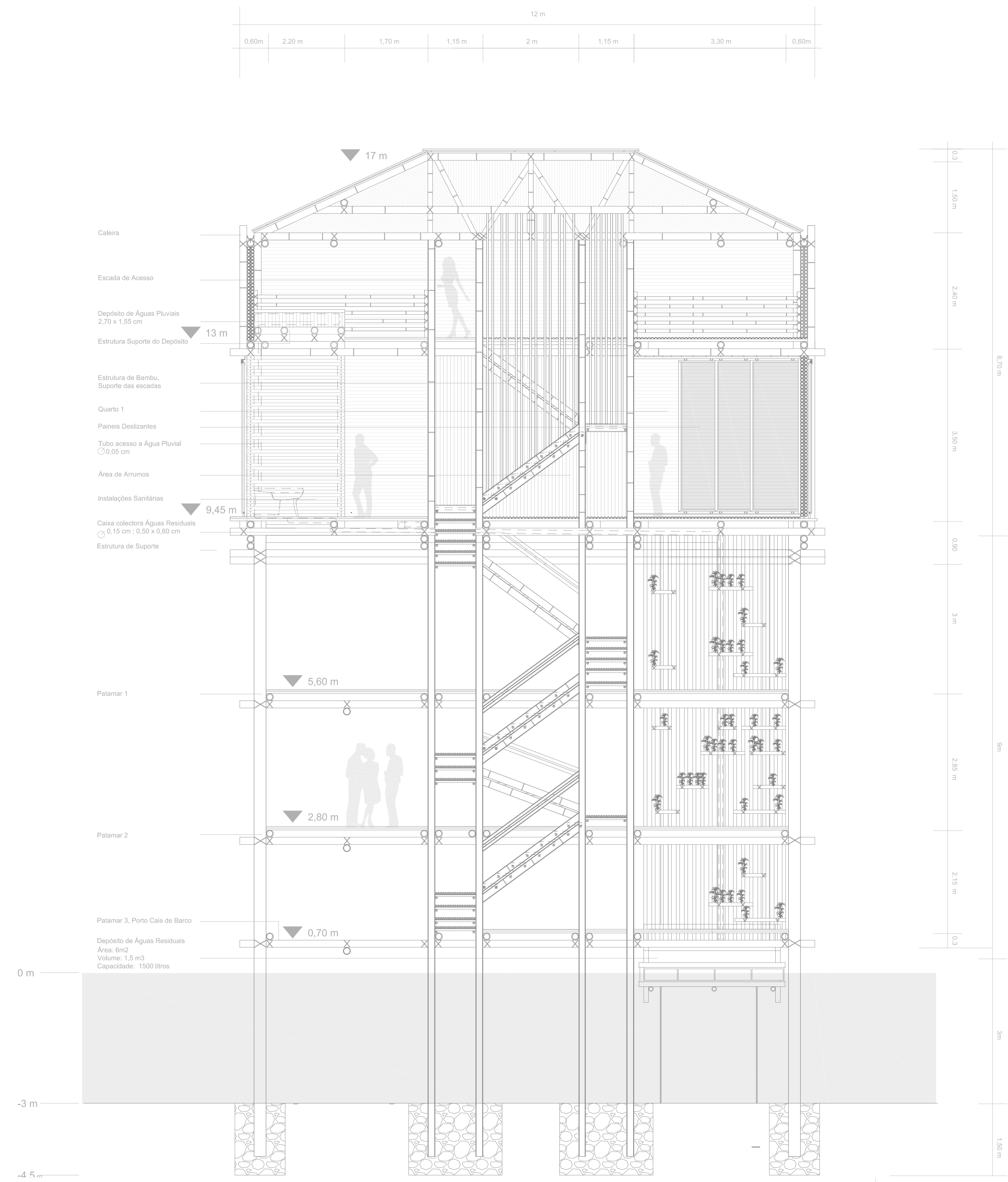
Corte B
