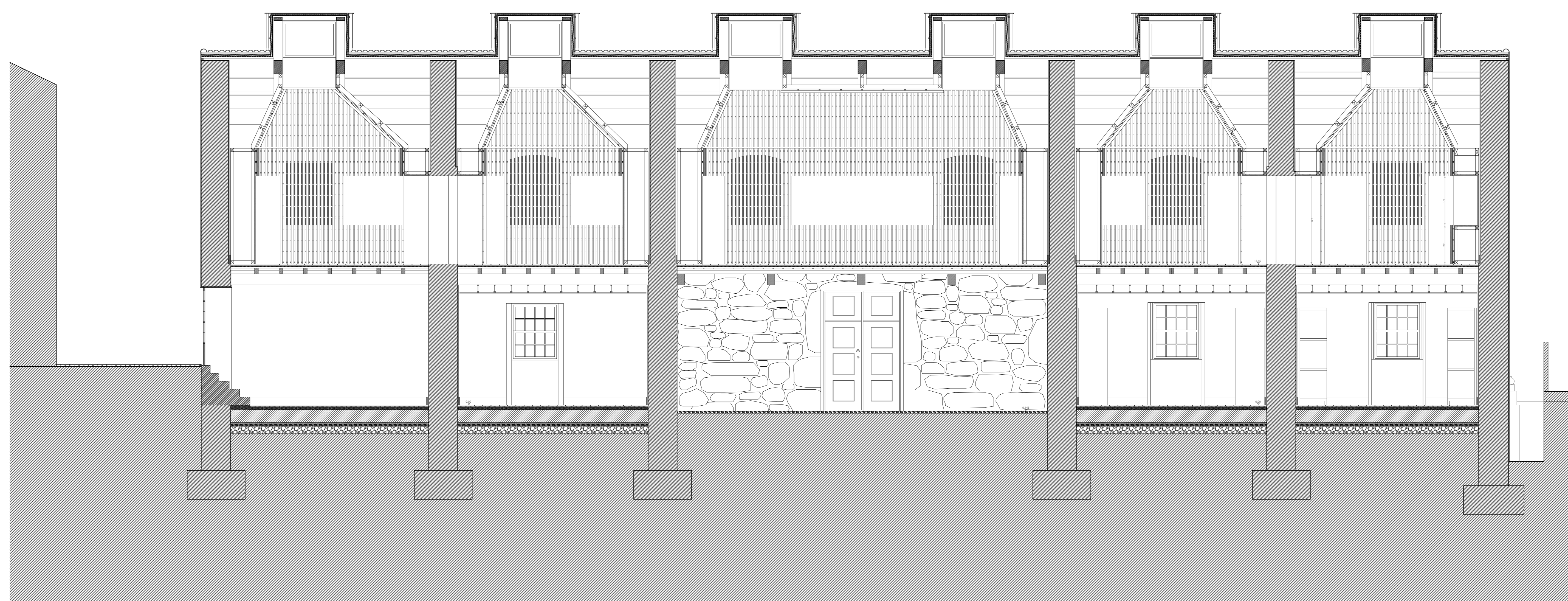
CORTE CC'
