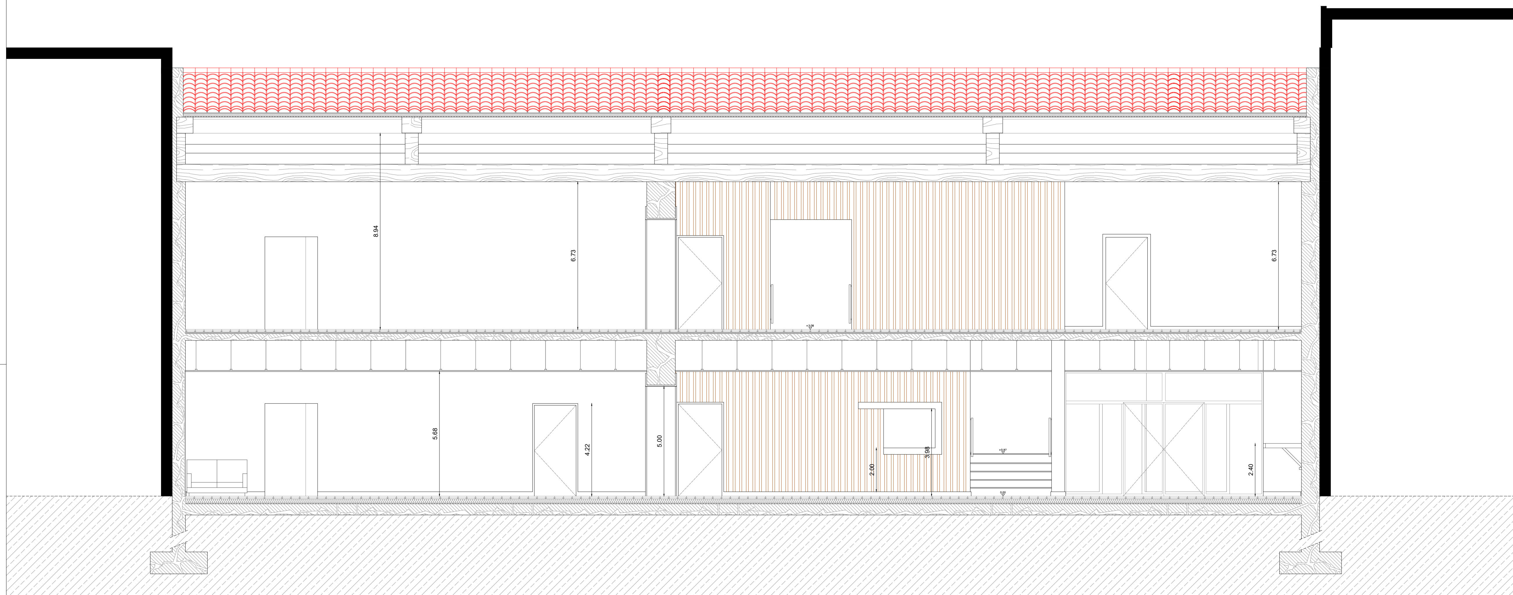
Corte C1
