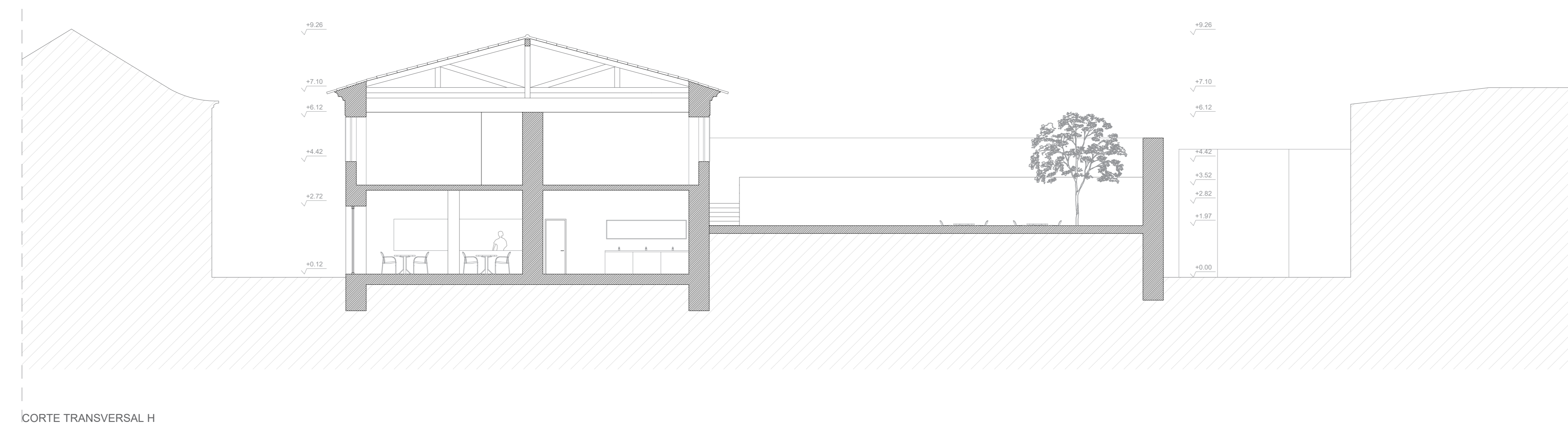
CORTE TRANSVERSAL H
