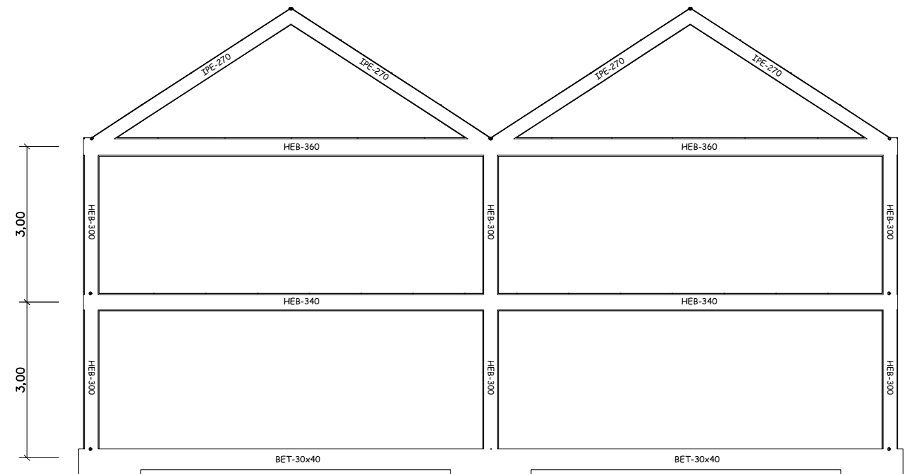
Pórticos 5/6
