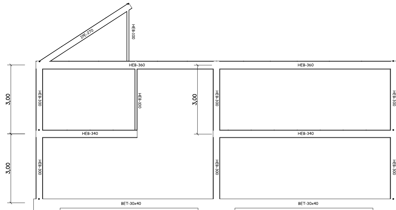
Pórticos 3/4
