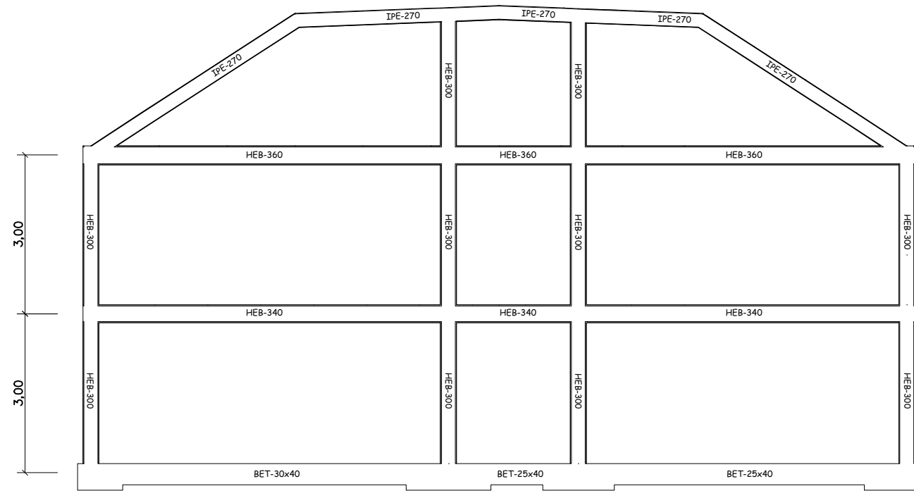
Pórtico 1
