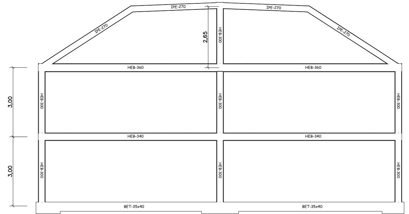
Pórtico 2
