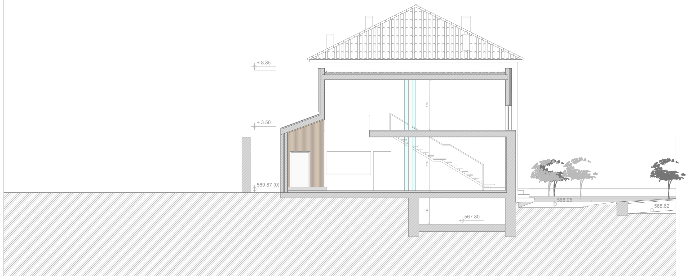
CORTE B
